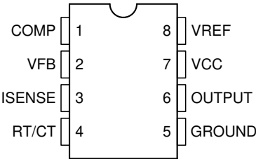
图 5-1. D、JG 和 P 封装 8 引脚 SOIC、CDIP 和 PDIP 顶视图
