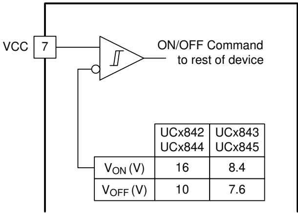
图 7-5. UVLO 阈值
