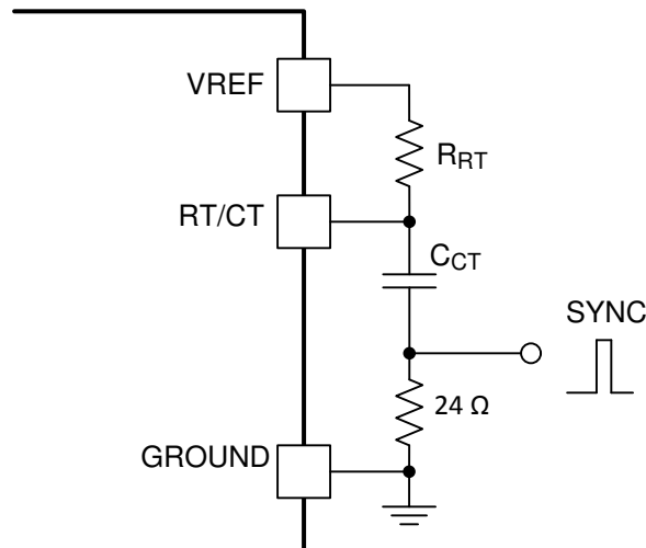
图 7-9. 同步振荡器
