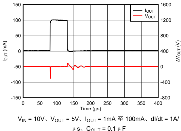
图 7-7. 负载瞬态特性 (M3 版本)
