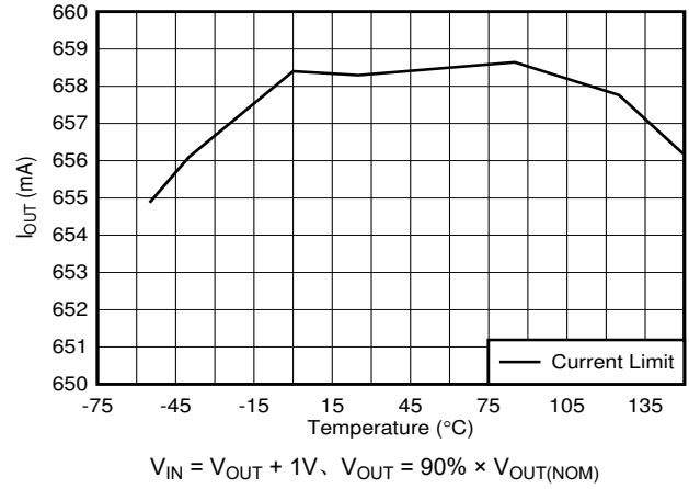
图 5-26. 输出电流限制与温度间的关系
