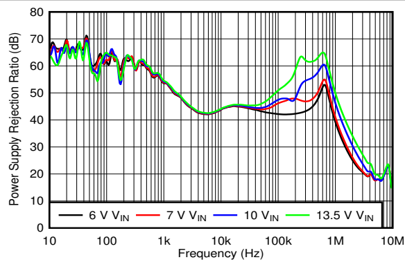
图 5-14. PSRR 与频率和 V_{IN} 间的关系
