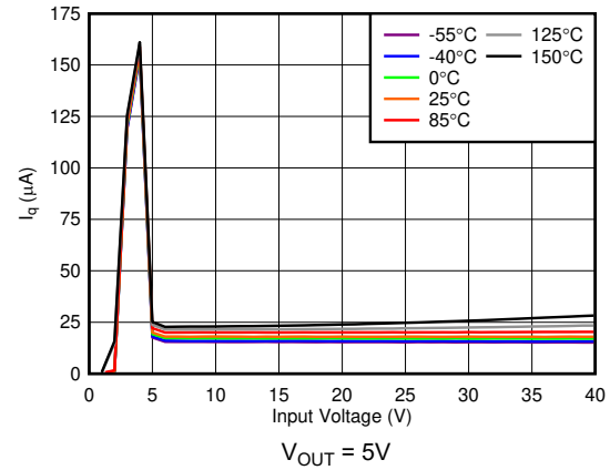
图 5-28. 静态电流 ( I_Q ) 与 V_{IN} 之间的关系
