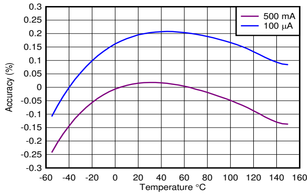
图 5-1. 精度与温度间的关系
