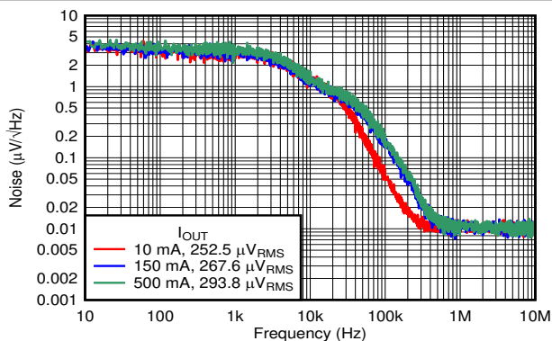
图 5-13. 噪声与频率间的关系
