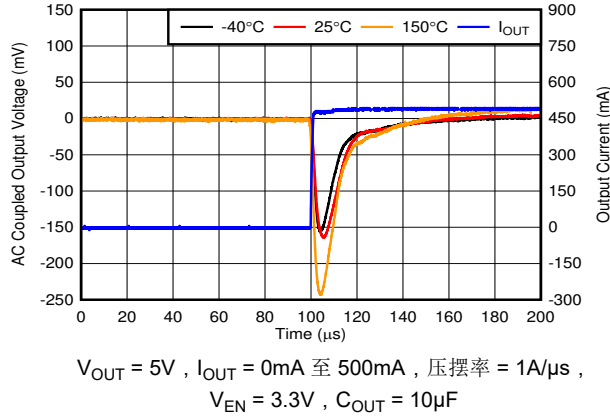
图 5-25. 负载瞬态, 500mA 上升沿无负载
