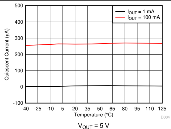
图 5-4. 静态电流与环境温度间的关系
