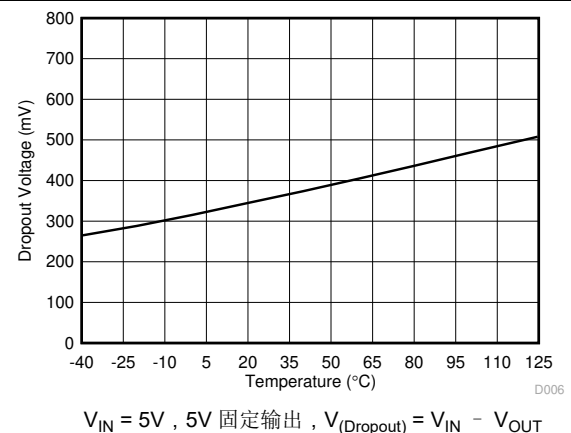
图 5-6. 压降电压与环境温度间的关系
