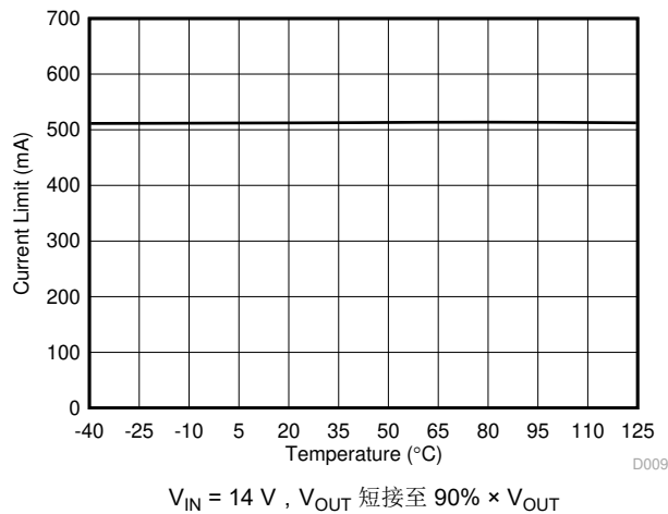
图 5-9. 输出电流限制与环境温度
