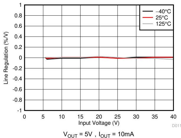
图 5-11. 线路调整
