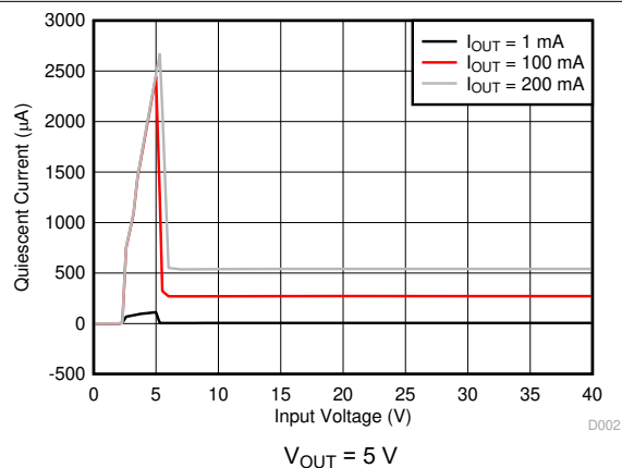
图 5-2. 静态电流与输入电压间的关系
