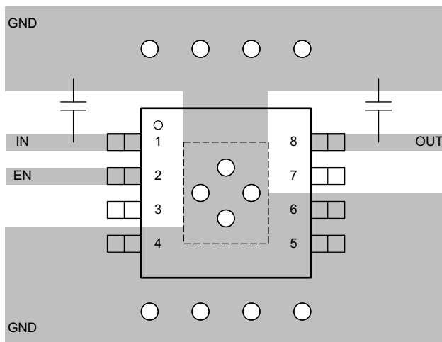
图 7-3. TPSB82-Q1 示例布局图
