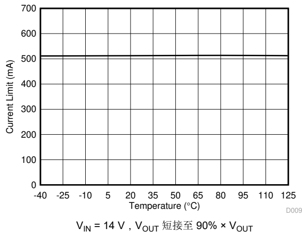
图 5-9. 输出电流限制与环境温度
