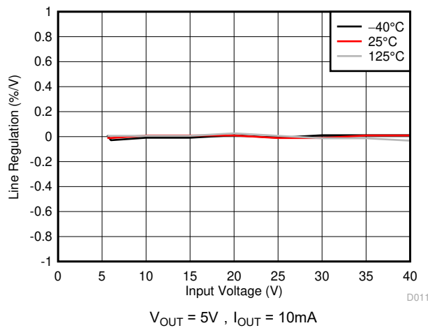
图 5-11. 线路调整
