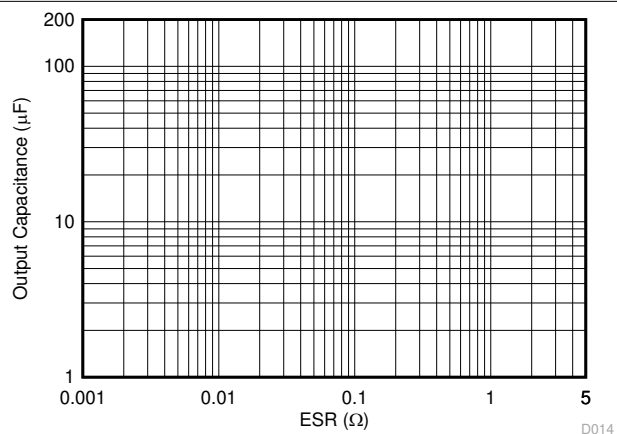
图 5-14. 输出电容与 ESR 稳定性间的关系
