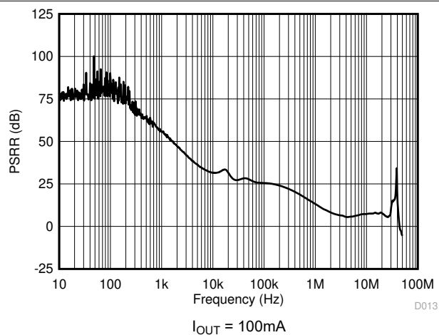
图 5-13. PSRR 与频率间的关系
