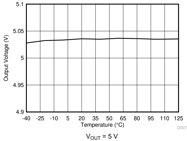
图 5-7. 输出电压与环境温度间的关系
