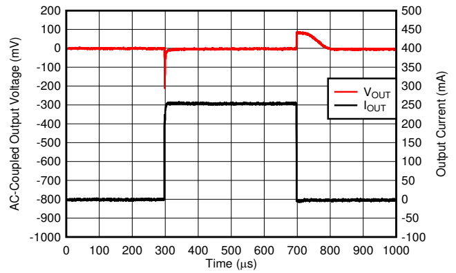
图 6-20. I_{OUT} Transient
