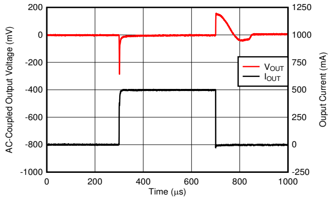
图 6-20. I_{OUT} Transient
