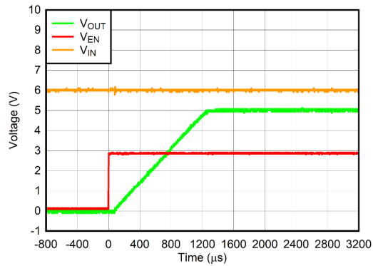
图 5-55. 在先施加 V_{IN} 后施加 V_{EN} 的情况下启动
