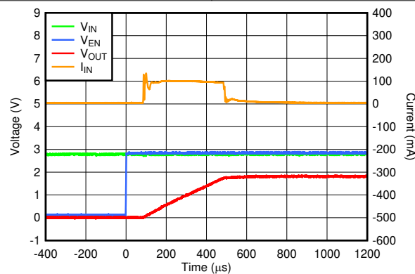
图 5-55. 在先施加 V_{IN} 后施加 V_{EN} 的情况下启动
