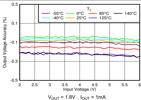
图 5-27. 输出精度与 V_{IN} 和温度间的关系
