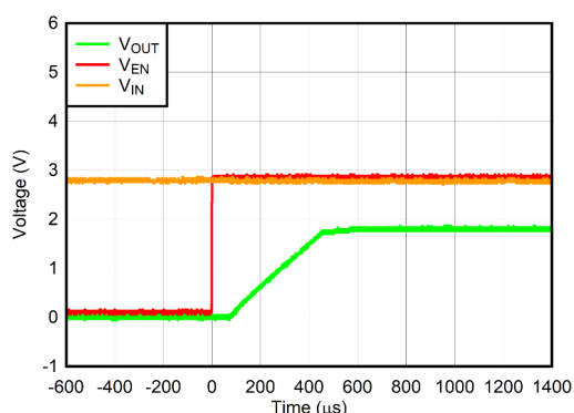
图 5-51. V_{EN} = V_{IN} 时的启动
