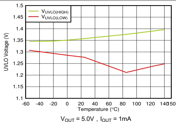
图 5-41. UVLO 上升和下降阈值与温度间的关系
