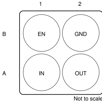
图 4-4. YCH 封装，4 引脚 DSBGA，0.35mm 间距 (底视图)
