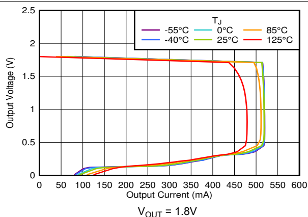
图 5-38. 折返电流限制与 I_{OUT} 和温度间的关系
