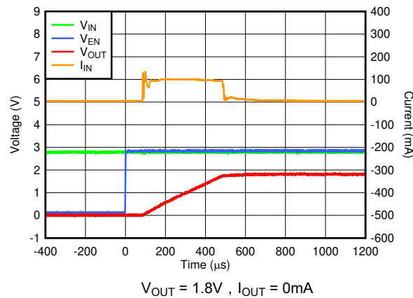
图 5-57. C_{OUT} = 22\mu\text{F} 时的启动浪涌电流
