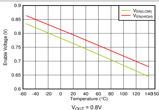
图 5-39. EN 高阈值和低阈值与温度间的关系
