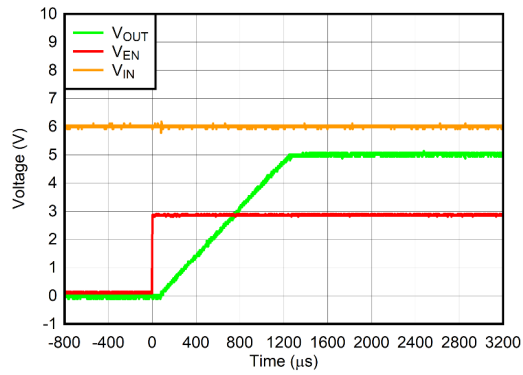
V_{OUT} = 5.0\text{V} , I_{OUT} = 200\text{mA} , C_{OUT} = 1\mu\text{F} 图 5-55. 在先施加 V_{IN} 后施加 V_{EN} 的情况下启动
