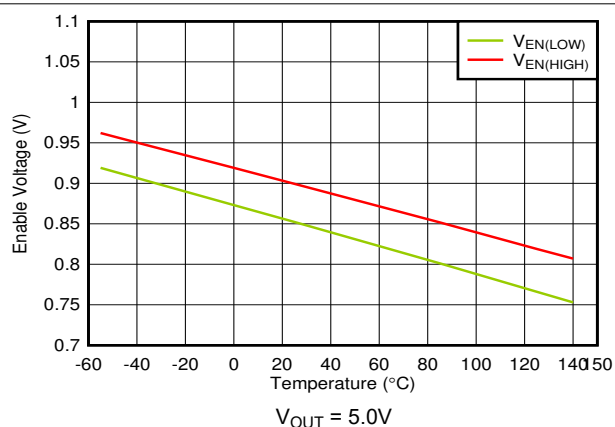
图 5-40. EN 高阈值和低阈值与温度间的关系
