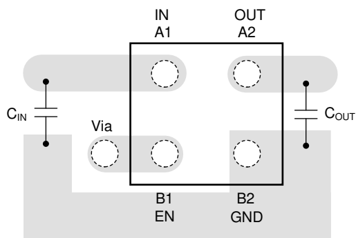
图 7-8. 采用 YCH 封装的布局示例
