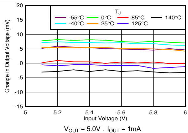
图 5-29. 线路调整与 V_{IN} 和温度之间的关系
