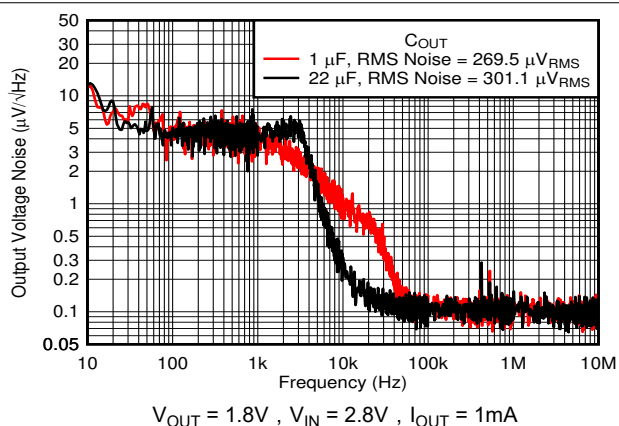
图 5-50. 输出噪声与频率和 C_{OUT} 间的关系
