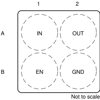
图 4-3. YCH 封装，4 引脚 DSBGA，0.35mm 间距 (顶视图)
