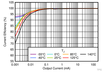
图 7-5. 电流效率与 I_{OUT} 和温度间的关系
