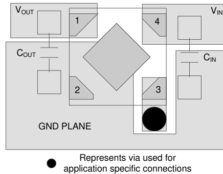
图 7-6. 采用 DQN 封装的布局示例
