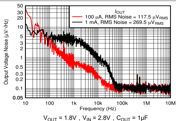
图 5-49. 输出噪声与频率和 I_{OUT} 间的关系
