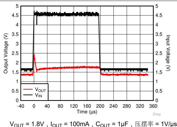
图 5-25. 从 1.5V 至 4.5V 的 V_{IN} 瞬态
