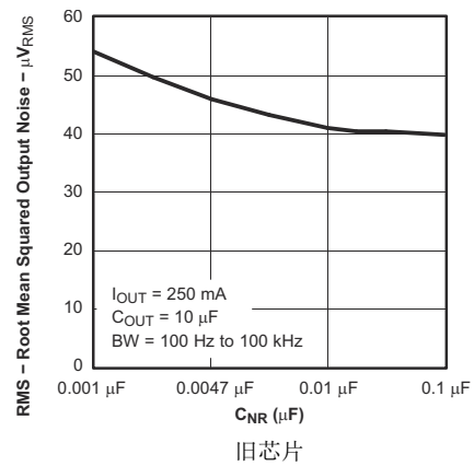
图 5-12. TPS79630 均方根输出噪声与旁路电容间的关系
