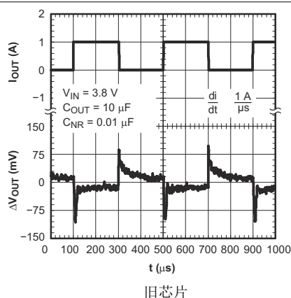
图 5-25. TPS79628 负载瞬态响应
