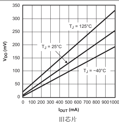
图 5-29. TPS79630 压降电压与输出电流间的关系
