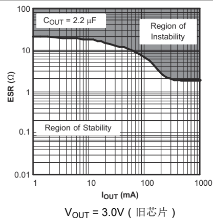
图 5-34. TPS795 典型稳定性区域等效串联电阻 (ESR) 与输出电流间的关系
