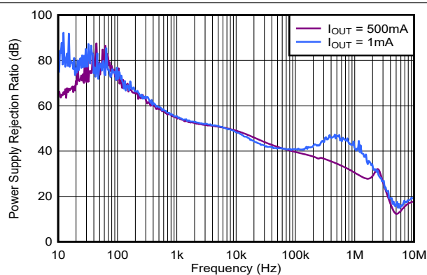
C_{OUT} = 2.2 \mu F 、 V_{OUT} = 3.3V (新芯片)
