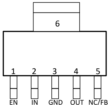
图 4-4. DCQ 封装，6 引脚 SOT-223 ( 顶视图，新芯片 )
