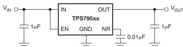
图 7-1. 典型应用电路
