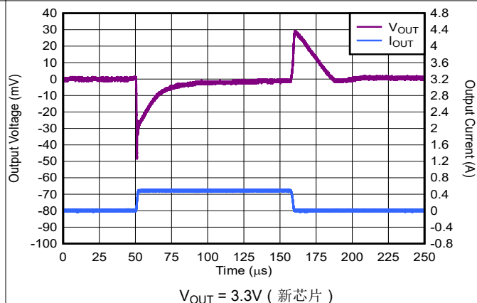
图 5-26. TPS795 负载瞬态响应
