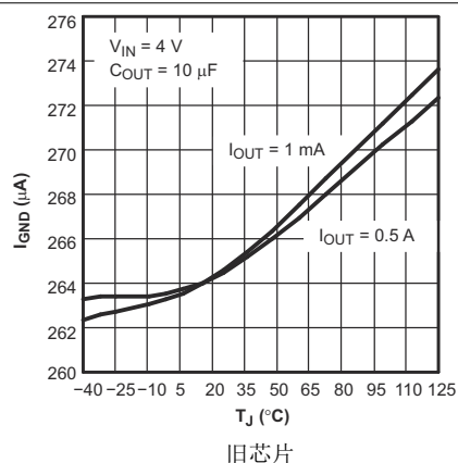
图 5-5. TPS795 接地电流与结温间的关系
