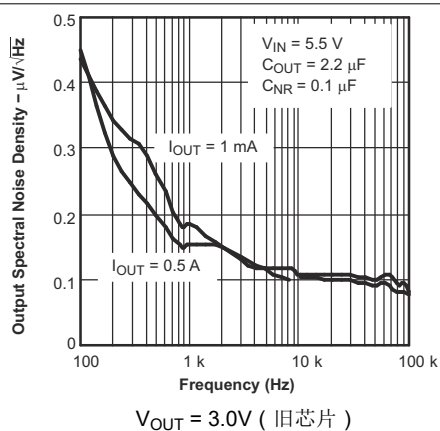
图 5-7. TPS795 输出频谱噪声密度与频率间的关系
