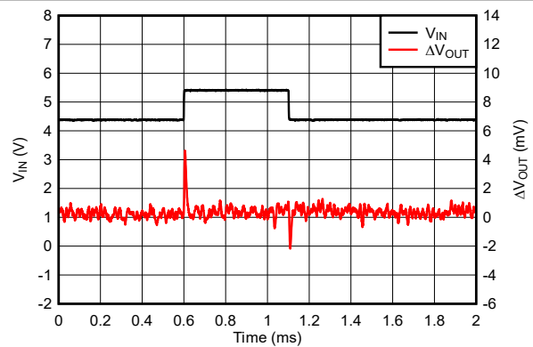
图 7-7. TPS77015 线路瞬态响应 (旧芯片)
