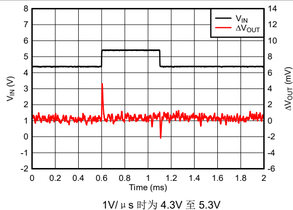
图 5-40. TPS76933 线路瞬态响应 (新芯片)
