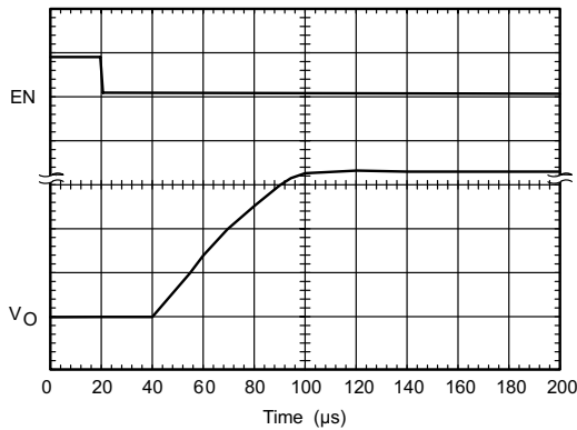
图 7-4. LDO 启动时间 (旧芯片)
