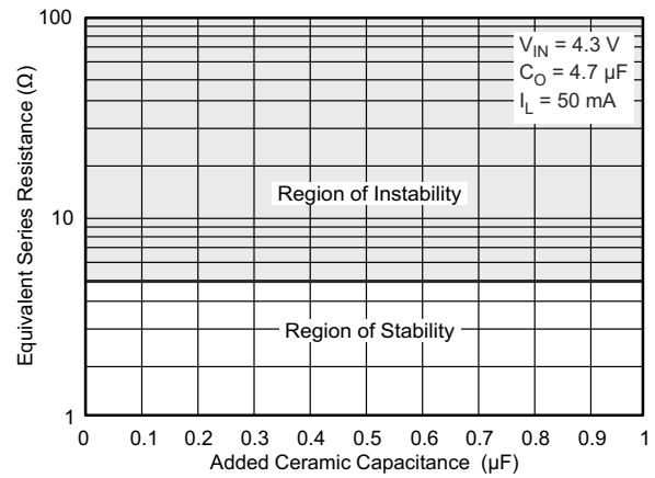
图 5-47. TPS77033 典型稳定性区域等效串联电阻 (ESR) 与添加的陶瓷电容间的关系 (旧芯片)
