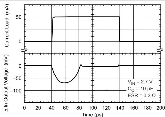
图 7-11. TPS77015 负载瞬态响应 (旧芯片)
