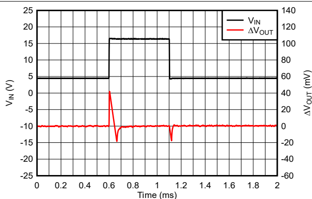
图 7-10. TPS77033 线路瞬态响应 (新芯片)
