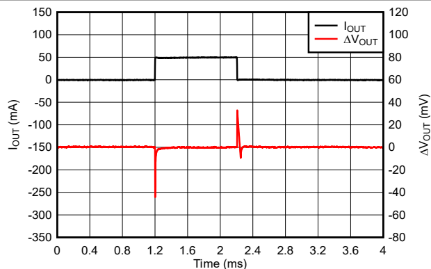
图 7-11. TPS77015 负载瞬态响应 (旧芯片)
