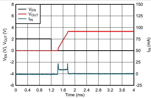
图 7-4. LDO 启动时间 (旧芯片)
