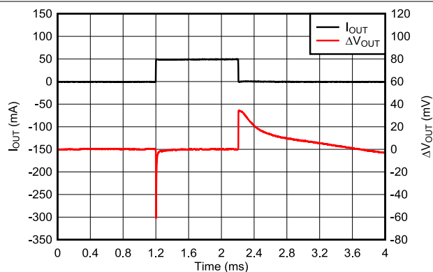
图 7-12. TPS77033 负载瞬态响应 (旧芯片)
