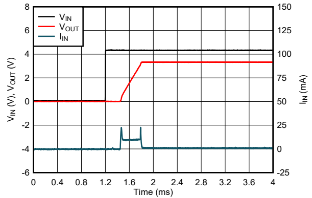
图 7-5. 采用输入电源时的 LDO 启动时间 (新芯片)
