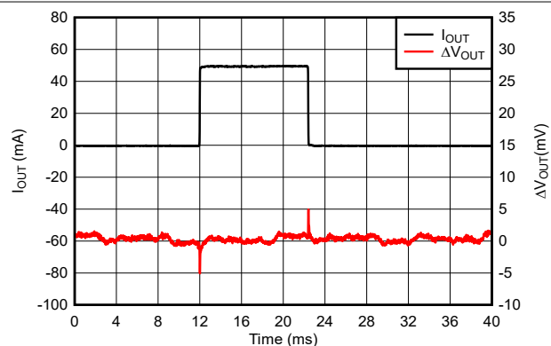
图 7-13. TPS77033 负载瞬态响应 (新芯片)
