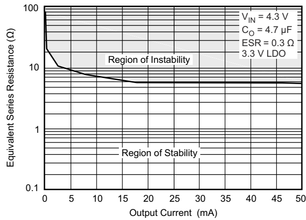
图 5-46. TPS77033 典型稳定性区域等效串联电阻 (ESR) 与输出电流间的关系 (旧芯片)
