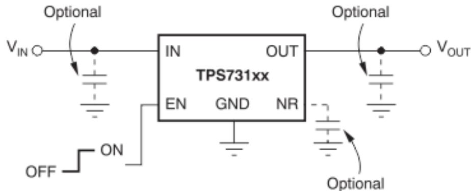
针对固定电压版本的典型应用电路
