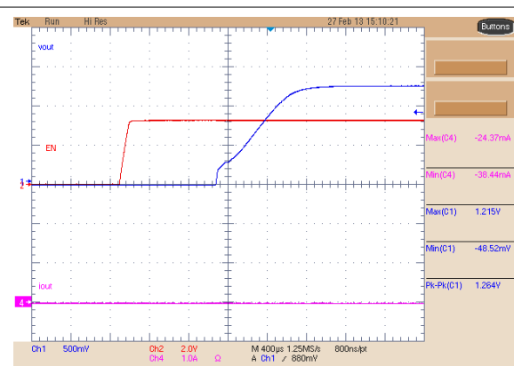
图 8-4. Buck 1 Soft-Start
