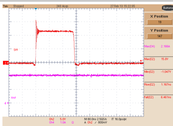
图 8-9. Buck 1 Switching Node, 2-A Load
