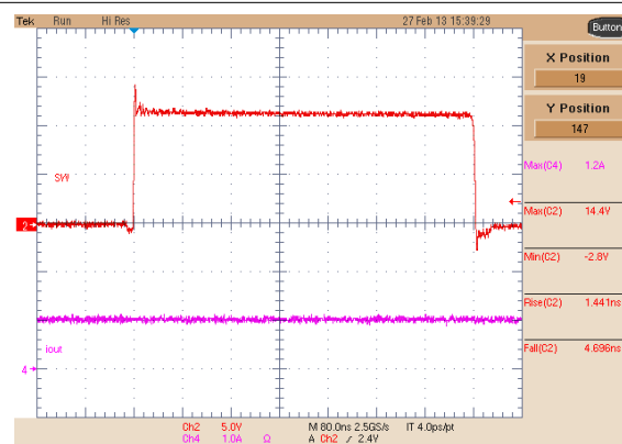
图 8-40. Buck 3 Switching Node, 1-A Load
