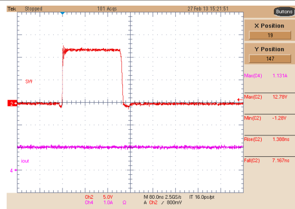
图 8-8. Buck 1 Switching Node, 1-A Load
