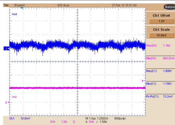
图 8-31. Buck 2 Ripple, 1-A Load
