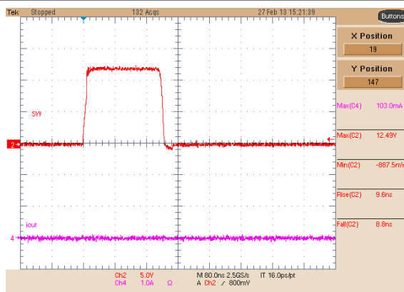
图 8-7. Buck 1 Switching Node, No Load
