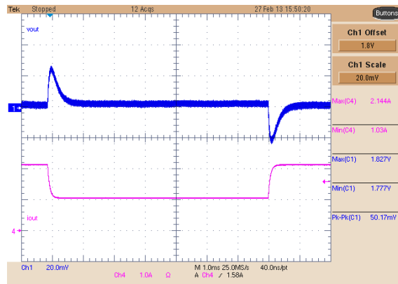
图 8-29. Buck 2 Dynamic Response, 1-A to 2-A Step
