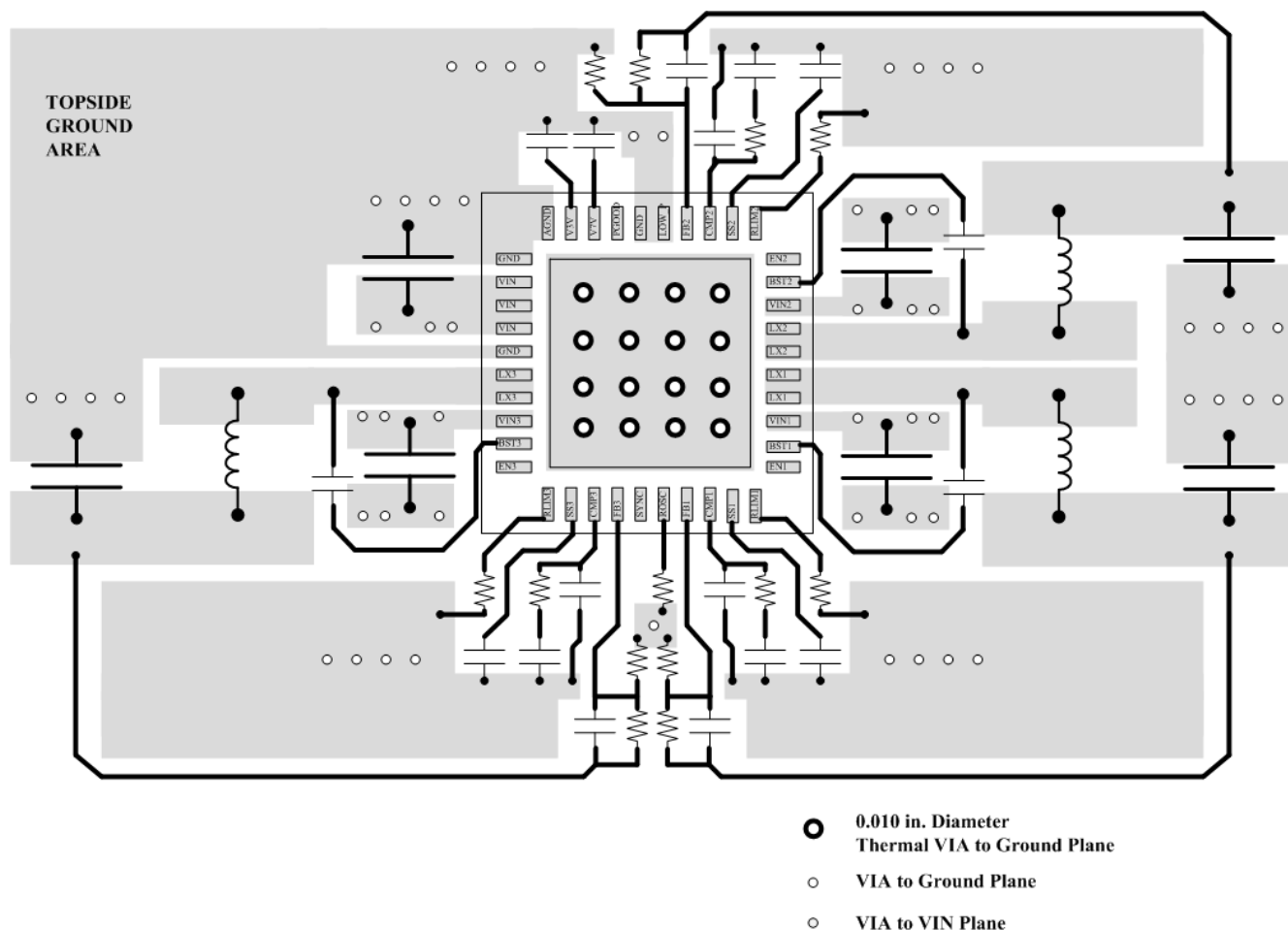
图 10-1. Layout Schematic
