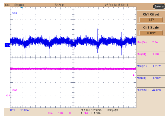
图 8-32. Buck 2 Ripple, 3-A Load
