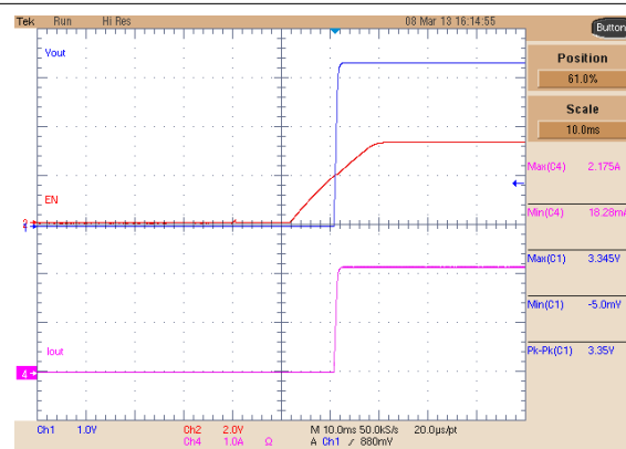
图 8-38. Buck 3 Soft-Start
