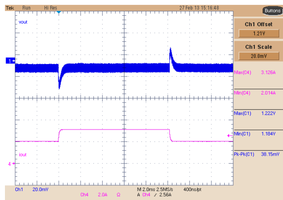
图 8-12. Buck 1 Dynamic Response, 2-A to 3-A Step
