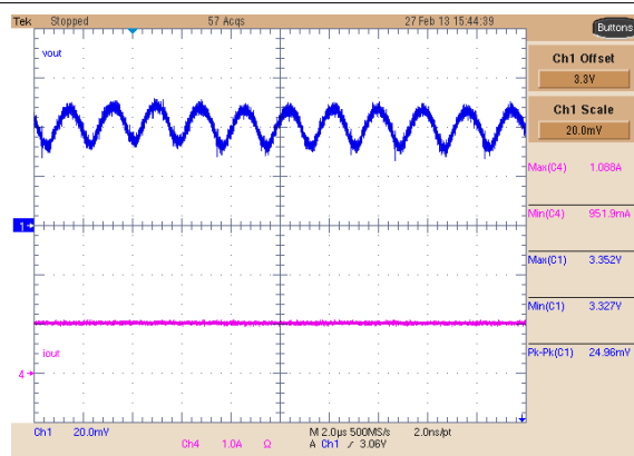
图 8-45. Buck 3 Ripple, 1-A Load
