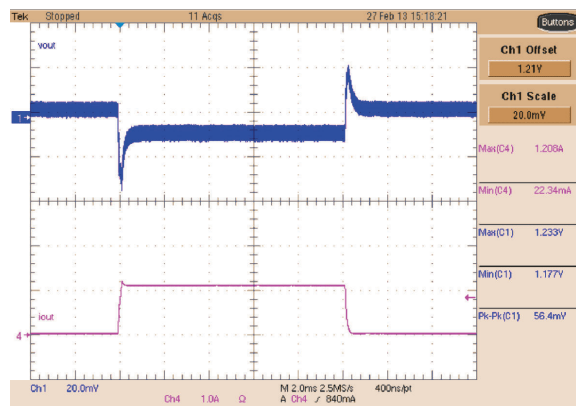
图 8-11. Buck 1 Dynamic Response, 0- to 1-A Step
