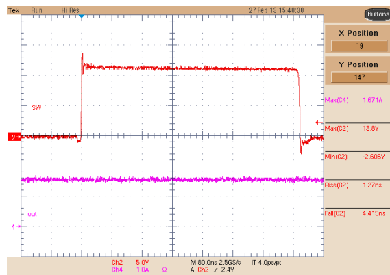
图 8-41. Buck 3 Switching Node, 1.5-A Load
