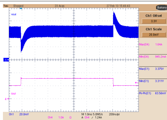
图 8-43. Buck 3 Dynamic Response, 1-A to 1.5-A Step
