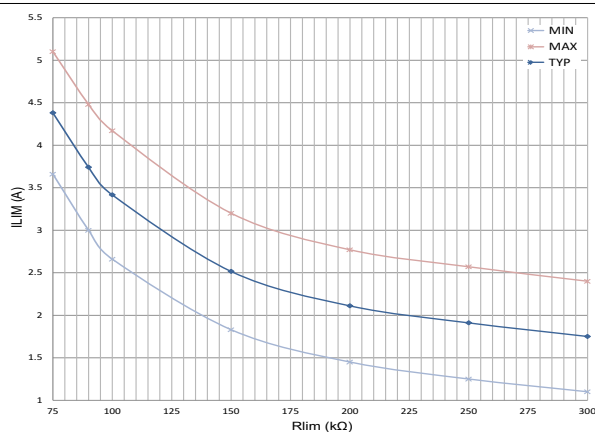
图 6-6. Current Limit V_{IN} = 12\text{ V} , f_{SW} = 500\text{ KHz}
