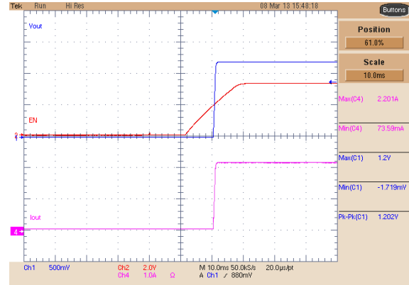
图 8-6. Buck 1 Soft-Start 2-A Load
