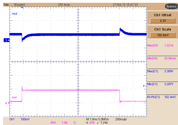
图 8-42. Buck 3 Dynamic Response, 0-A to 1-A Step
