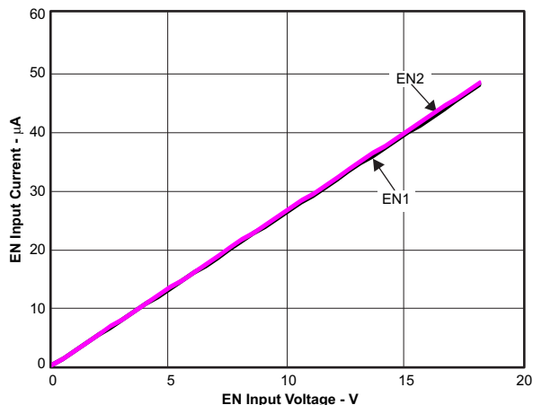
Figure 3. EN Current vs EN Voltage ( V_{IN}=12\text{ V} )
