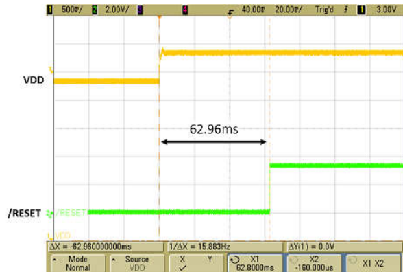
图 7-4. Reset Delay
