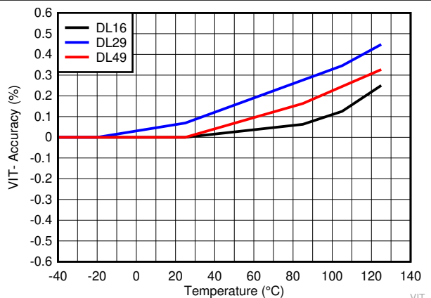
图 6-7. TPS3840DLXX 负向输入阈值精度随温度变化曲线
