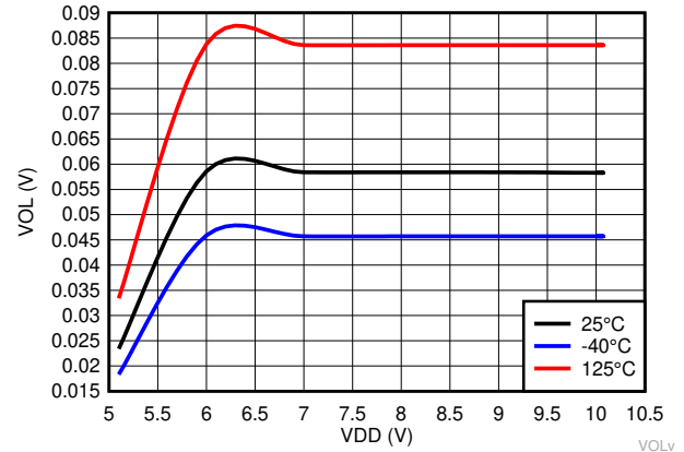
图 6-21. TPS3840PH49 的低电平输出电压与 V_{\text{DD}} 间的关系
