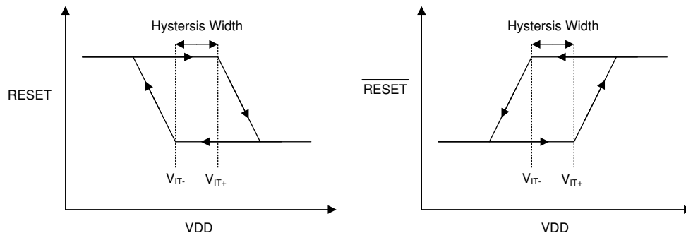
图 7-1. 迟滞图
