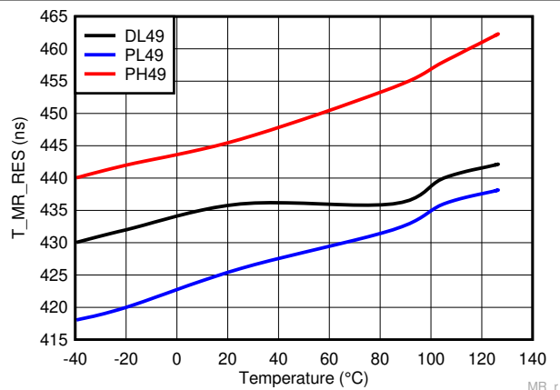
图 6-40. 从 \overline{\text{MR}} 置为有效到复位的传播延时时间随温度变化曲线
