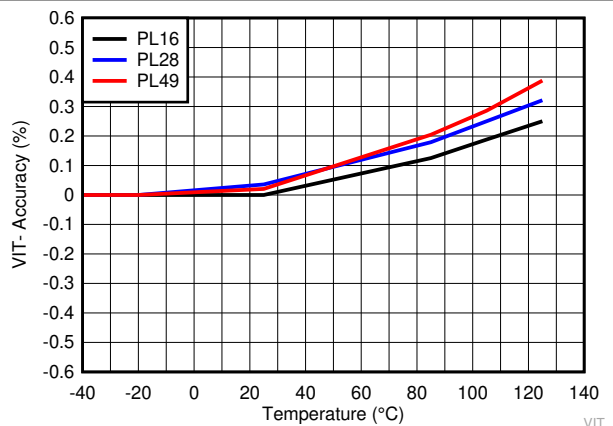
图 6-8. TPS3840PLXX 负向输入阈值精度随温度变化曲线
