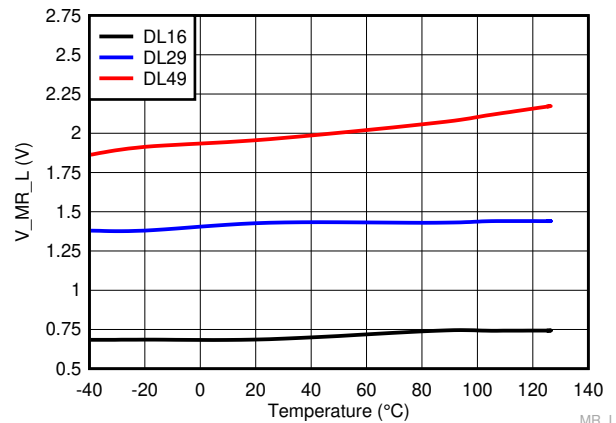
图 6-26. TPS3840DLXX 的手动复位逻辑低电平电压阈值随温度变化曲线
