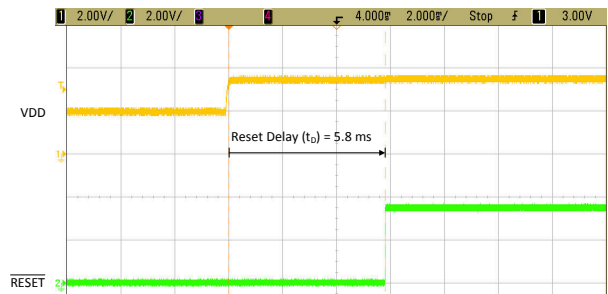
图 8-8. TPS3840EVM 使用 0.01 \mu F 电容器时的 \overline{RESET} 延时时间 ( t_D )
