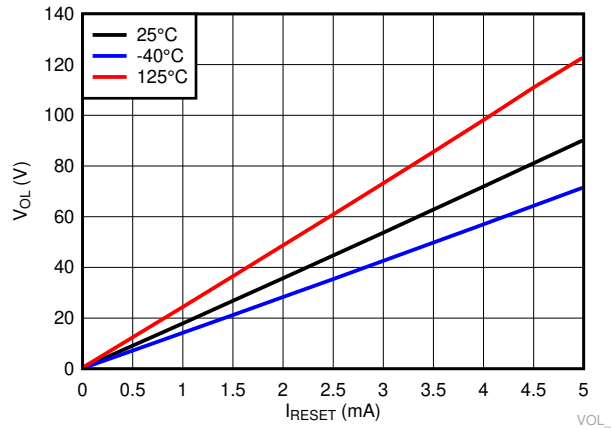
图 6-16. TPS3840DL49 的低电平输出电压与 I_{\text{RESET}} 间的关系
