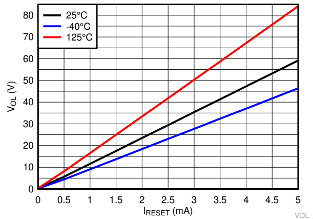
图 6-20. TPS3840PH49 的低电平输出电压与 I_{\text{RESET}} 间的关系
