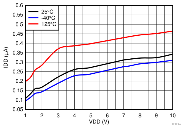
图 6-6. TPS3840PH49 的电源电流与电源电压间的关系
