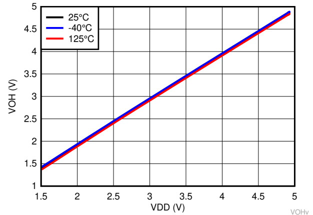
图 6-25. TPS3840PH49 的高电平输出电压随温度变化曲线
