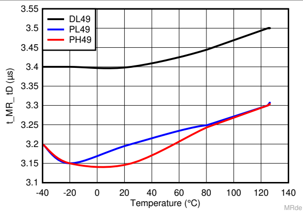
图 6-41. 从 \overline{\text{MR}} 释放为置为无效到复位的传播延时时间随温度变化曲线
