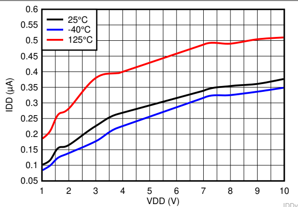
图 6-5. TPS3840PL49 的电源电流与电源电压间的关系
