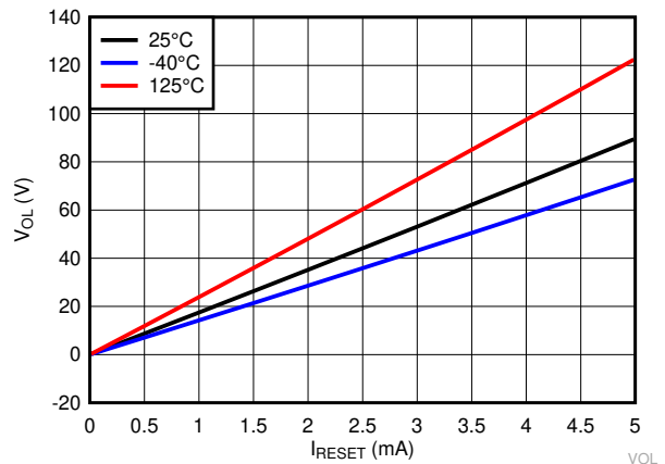
图 6-18. TPS3840PL49 的低电平输出电压与 I_{\text{RESET}} 间的关系
