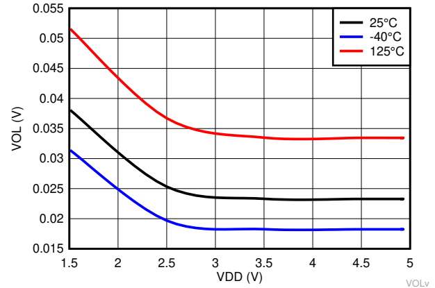
图 6-17. TPS3840DL49 的低电平输出电压与 V_{\text{DD}} 间的关系
