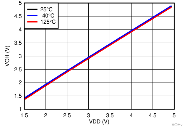
图 6-23. TPS3840PL49 的高电平输出电压随温度变化曲线
