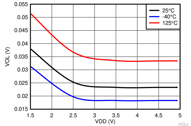
图 6-19. TPS3840PL49 的低电平输出电压与 V_{\text{DD}} 间的关系
