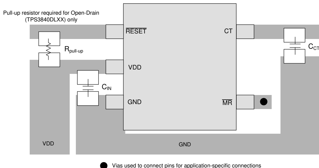
图 8-10. TPS3840 建议布局
