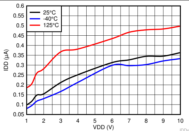
图 6-4. TPS3840DL49 的电源电流与电源电压间的关系
