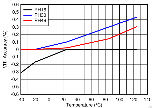
图 6-9. TPS3840PHXX 负向输入阈值精度随温度变化曲线
