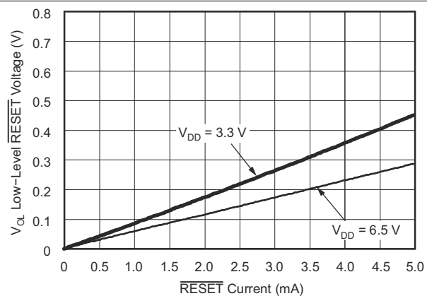
图 6-8. 低电平 \overline{\text{RESET}} 电压与 \overline{\text{RESET}} 电流间的关系
