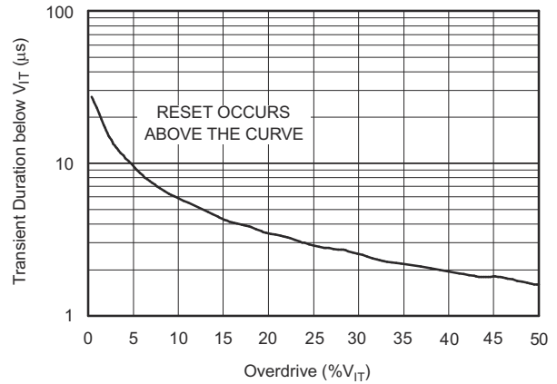
图 6-5. SENSE 上的最大瞬态持续时间与 SENSE 阈值过驱电压间的关系
