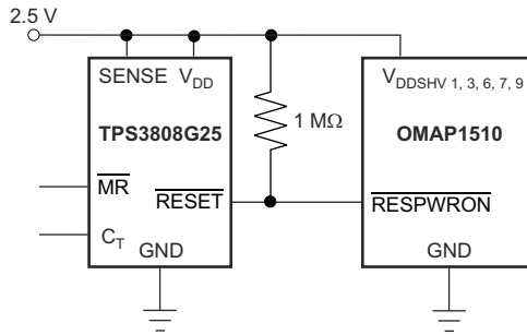
图 8-1. TPS3808 与 OMAP™ 处理器配合使用的典型应用
