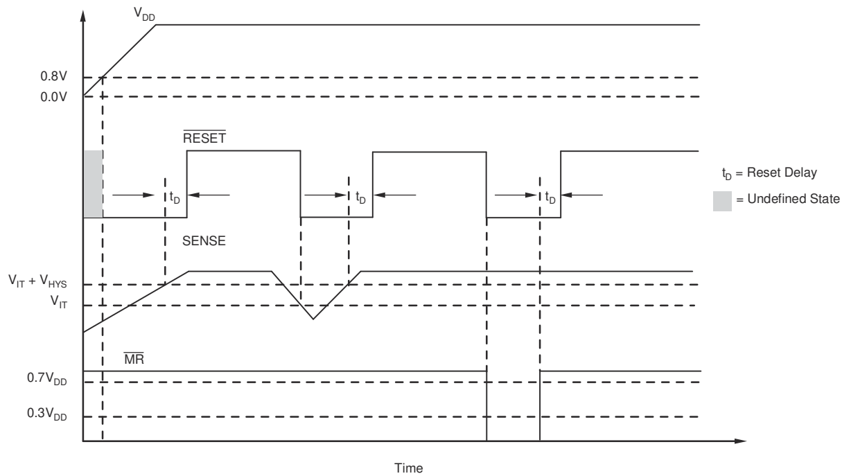
图 6-1. 显示 \overline{MR} 和 SENSE 复位时序的 TPS3808 时序图
