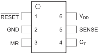
图 5-1. DBV 封装 6 引脚 SOT-23 顶视图
