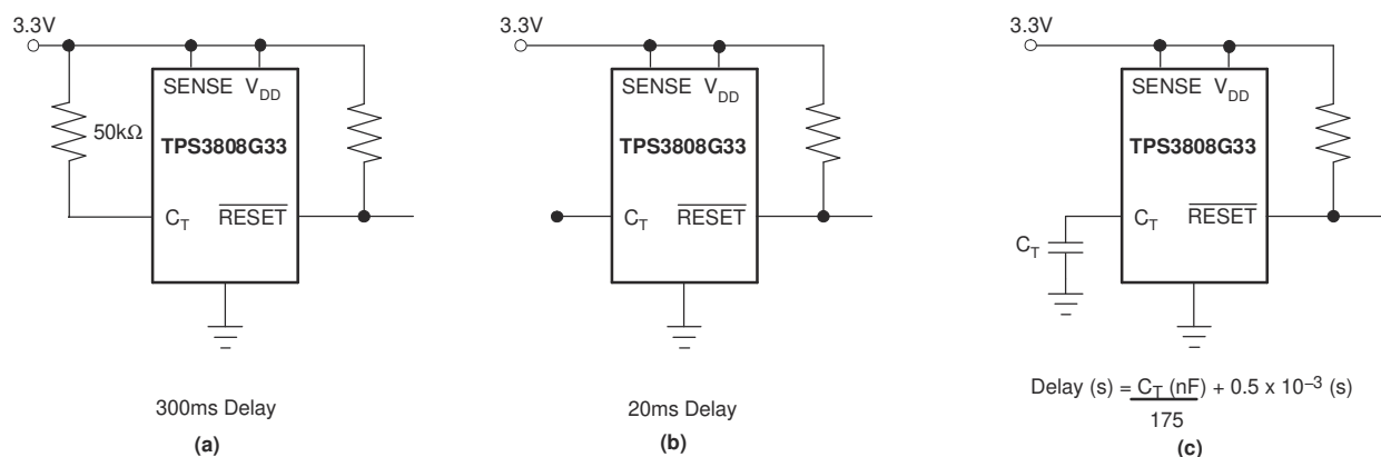
图 7-2. 用于设置 \overline{\text{RESET}} 延迟时间的配置
