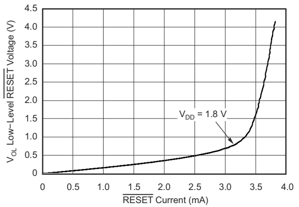
图 6-7. 低电平 RESET 电压与 RESET 电流间的关系
