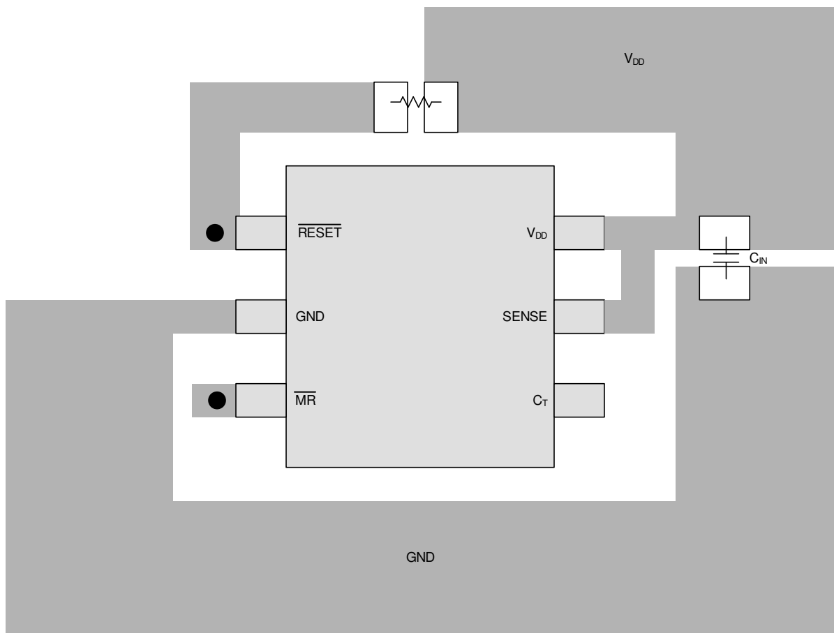
图 8-3. 20ms 延迟的布局示例
