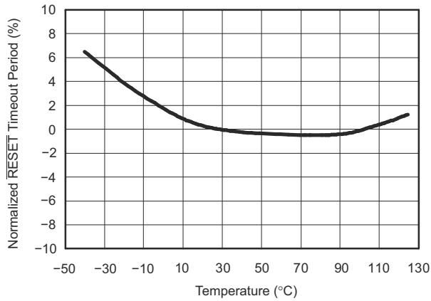
图 6-4. 标准化 RESET 超时周期与温度间的关系 ( C_T = \text{开路} , C_T = V_{DD} , C_T = \text{任意} )
