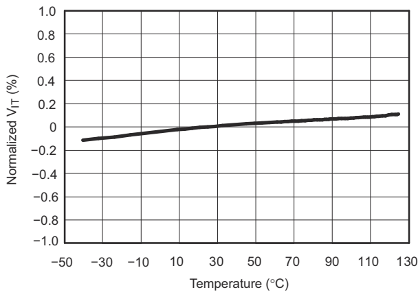
图 6-6. 标准化检测阈值电压 ( V_{IT} ) 与温度间的关系
