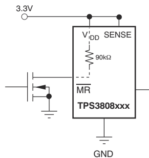
图 7-4. 当 \overline{\text{MR}} 信号没有进入 V_{DD} 时，使用外部 MOSFET 来尽可能降低 I_{DD}
