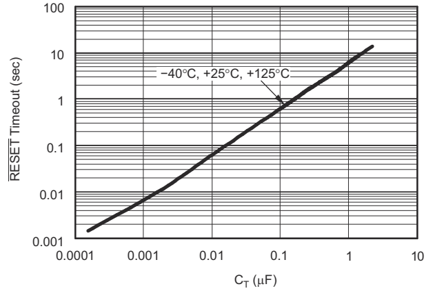
图 6-3. RESET 超时周期与 C_T 间的关系
