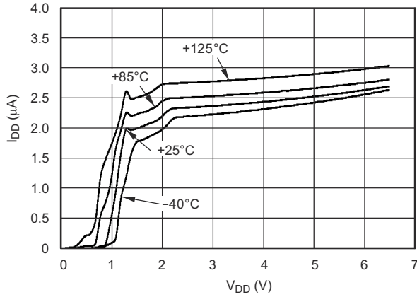
图 6-2. 电源电流与电源电压间的关系
