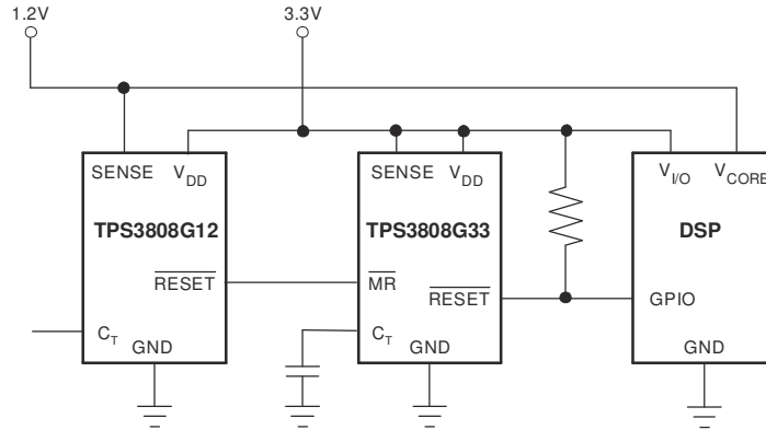
图 7-3. 使用 \overline{\text{MR}} 监控多个系统电压
