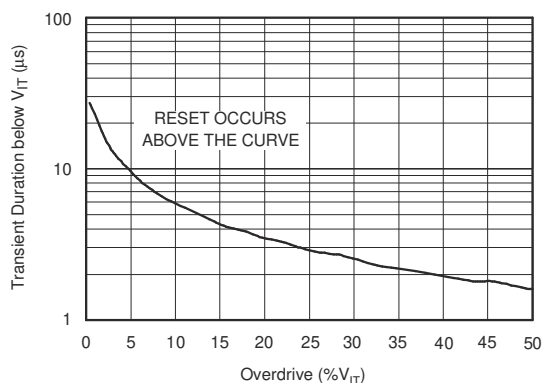
图 8-2. SENSE 上的最大瞬态持续时间与 SENSE 阈值过驱电压间的关系
