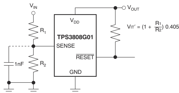
图 7-1. 使用 TPS3808G01 监控用户定义的阈值电压
