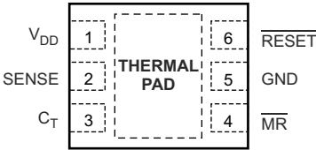
图 5-2. DRV 封装 6 引脚 (2.00mm × 2.00mm) WSON (带散热焊盘) 顶视图
