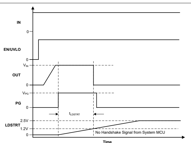
图 7-7. 失败的 LDSTRT 握手
