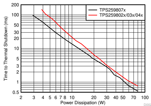
图 6-23. 热关断图 - 浪涌/过载
