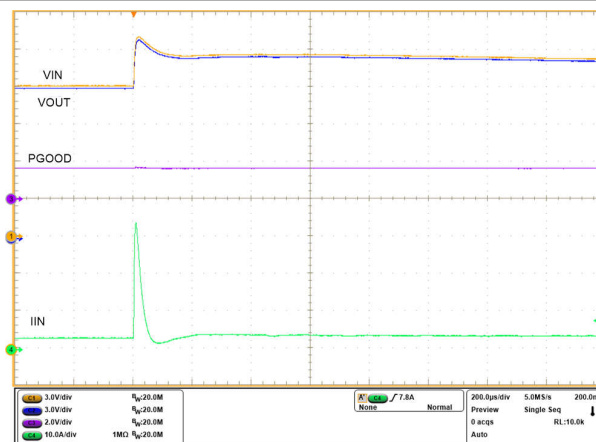
图 6-33. 电源线瞬态抗扰度 - 输入电压阶跃
