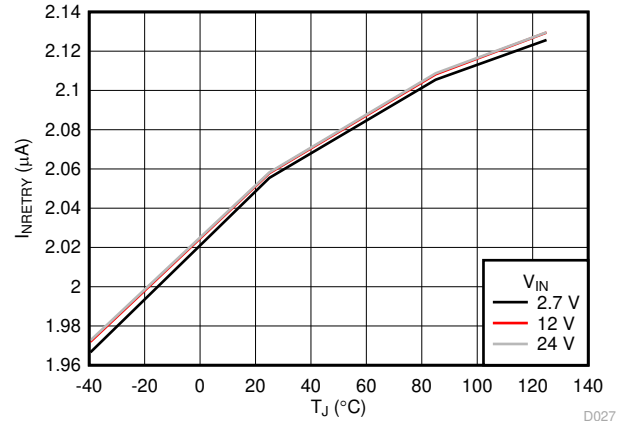
图 6-20. NRETRY 偏置电流与温度间的关系
