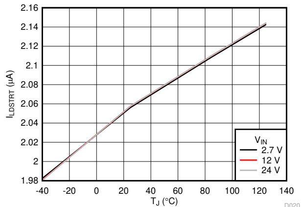
图 6-15. LDSTRT 充电电流与温度间的关系
