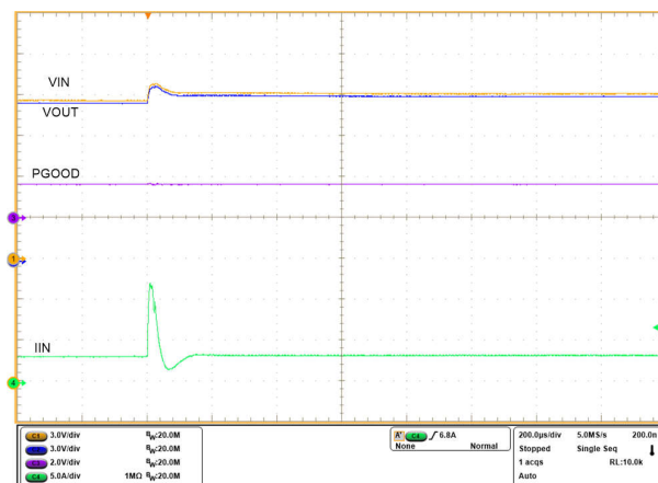
图 6-32. 导通时输出硬短路 (放大图)
