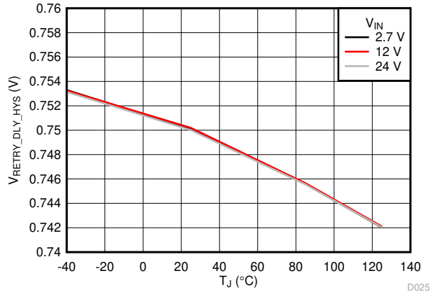
图 6-19. RETRY_DLY 振荡器磁滞与温度间的关系
