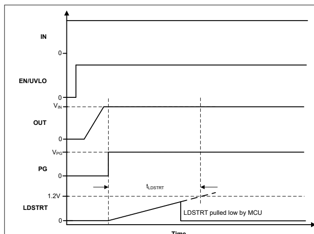
图 7-6. 成功的 LDSTRT 握手
