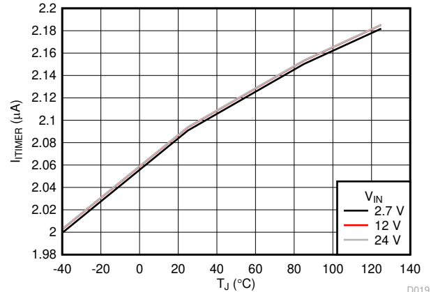
图 6-14. ITIMER 放电电流与温度间的关系
