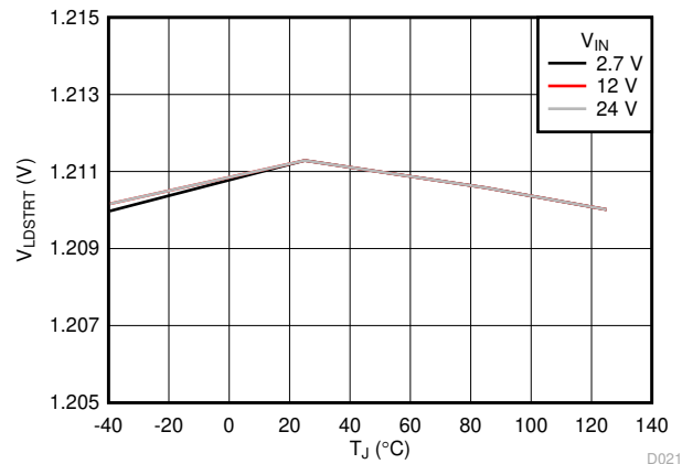
图 6-16. LDSTRT 阈值电压与温度间的关系
