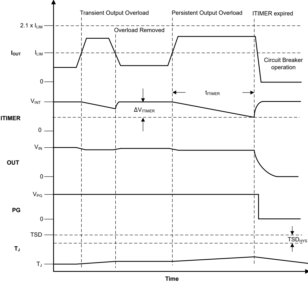
图 7-3. 断路器响应
