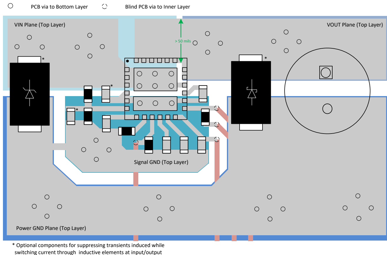
图 8-22. TPS25980 示例 PCB 布局
