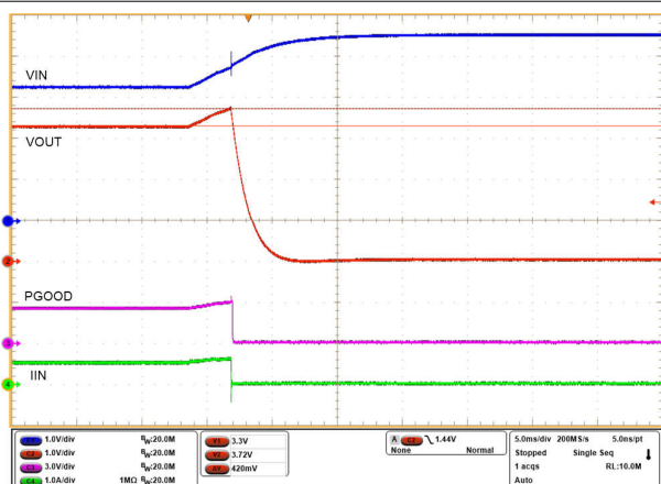
图 8-19. 采用 TPS2598020 器件的 3.7V 过压切断
