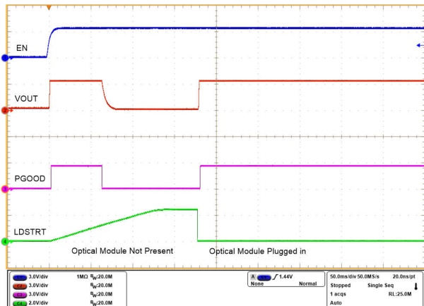
图 8-15. 插入光学模块时的输出电压曲线
