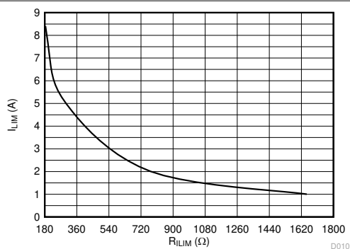
图 6-10. 输出电流限制 ( I_{LIM} ) 与 R_{LIM} 间的关系
