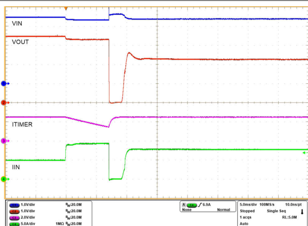
图 8-17. 具有 6ms 瞬态过流消隐间隔的断路器；器件在电流限制模式下重新启
