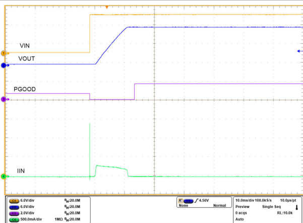
图 6-24. 热插拔
