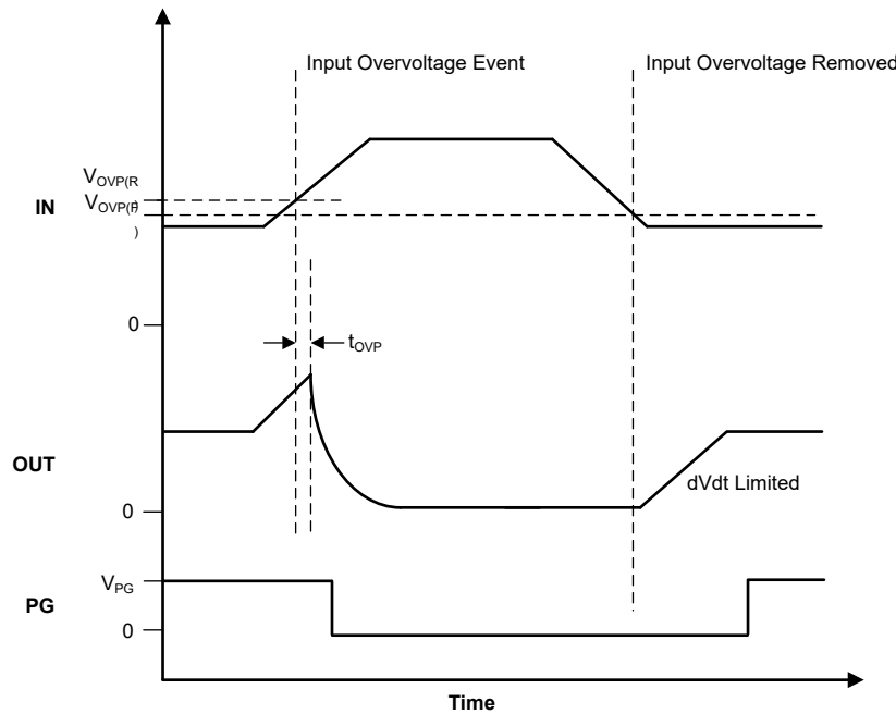
图 7-2. 过压响应
