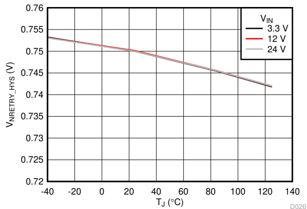
图 6-21. NRETRY 振荡器磁滞与温度间的关系
