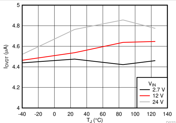
图 6-17. DVDT 充电电流与温度间的关系
