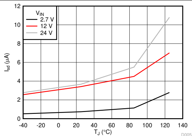
图 6-9. 深度关断电流与温度间的关系
