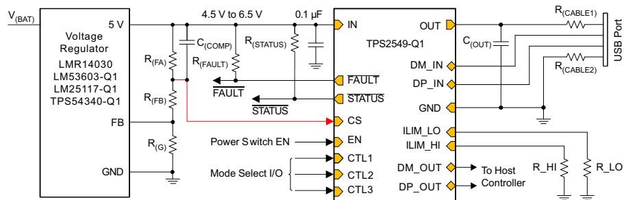
简化原理图
