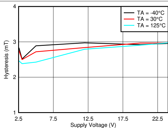
图 7-11. Hysteresis_X 与 V CC
