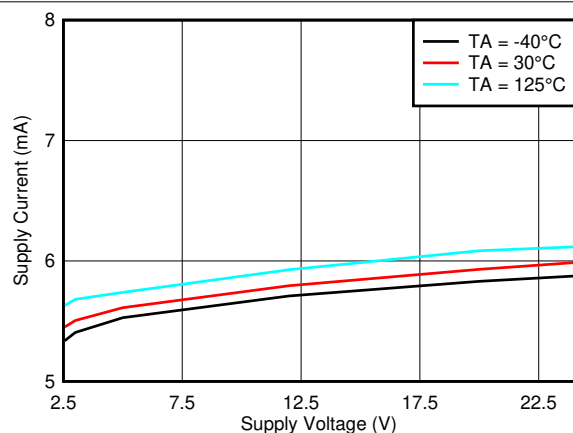
图 7-37. 电源电流与 V_{CC}
