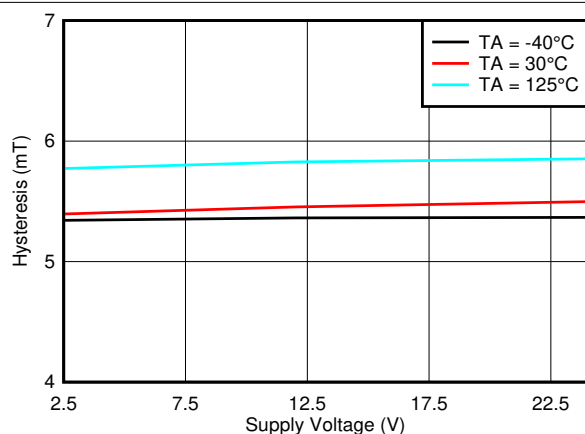
图 7-55. Hysteresis_Y 与 V CC
