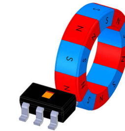
图 8-10. ZY 外边缘 1
