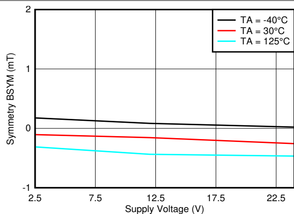
图 7-59. B_{SYM(X)} 与 V_{CC}
