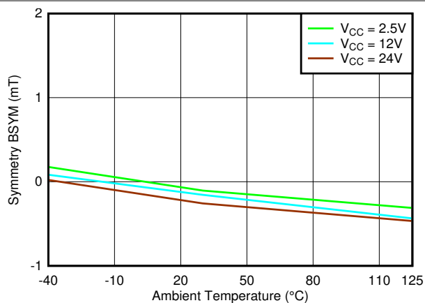
图 7-60. B_{SYM(X)} 与温度
