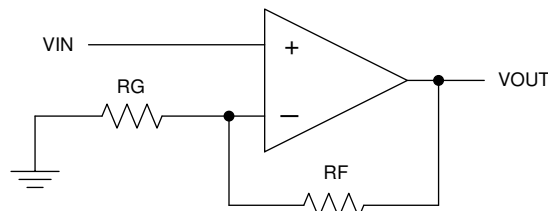
图 7-3. 原理图表示
