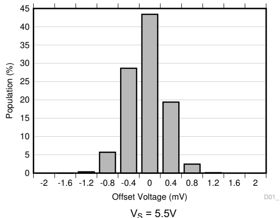
图 6-1. 失调电压分布直方图
