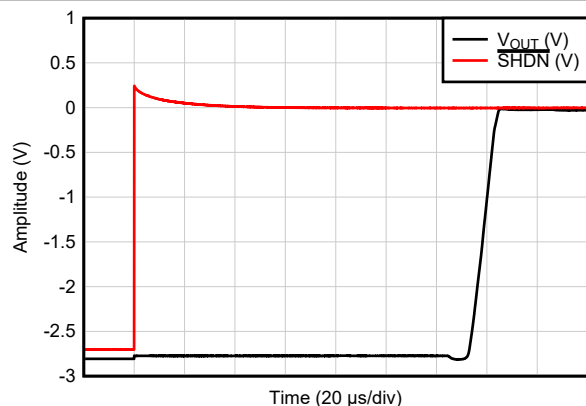
图 6-43. 放大器启用响应
