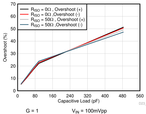
图 6-29. 小信号过冲与容性负载间的关系
