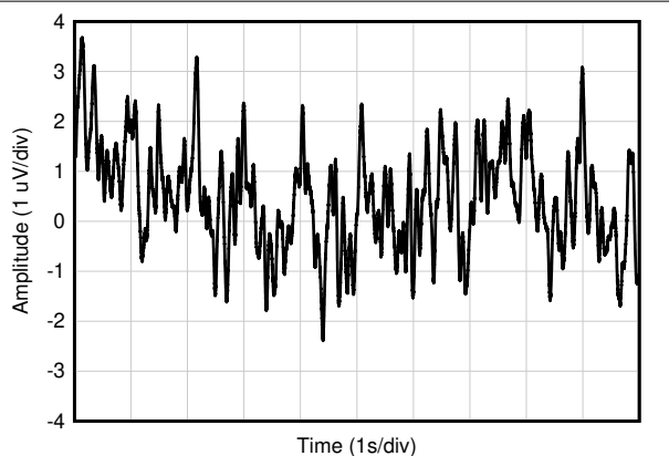
图 6-21. 0.1Hz 至 10Hz 时域电压噪声
