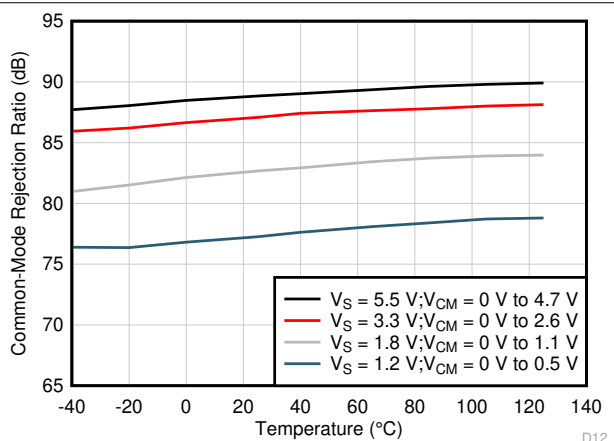
图 6-20. 直流 CMRR 与温度间的关系
