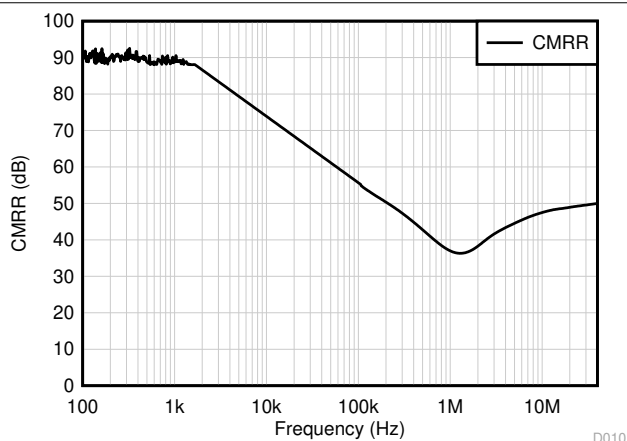
图 6-19. CMRR 与频率间的关系
