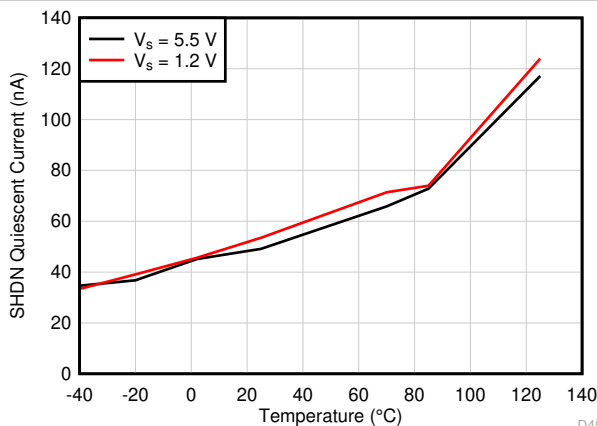
图 6-42. 关断模式静态电流与温度间的关系
