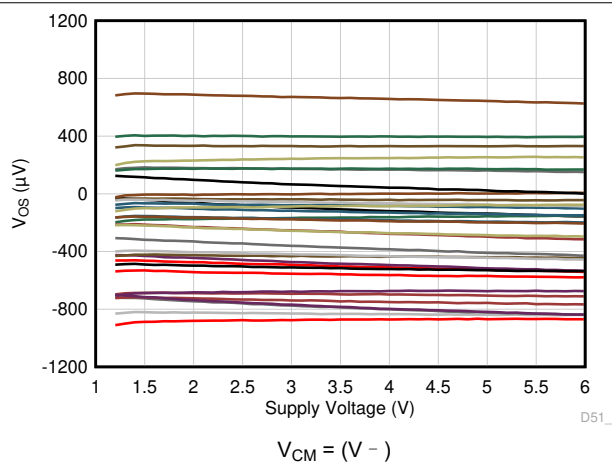
图 6-7. 偏移电压与电源电压间的关系
