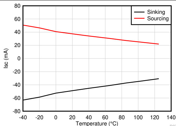
图 6-40. 短路电流与温度间的关系
