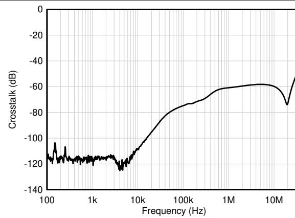
图 6-46. 通道分离
