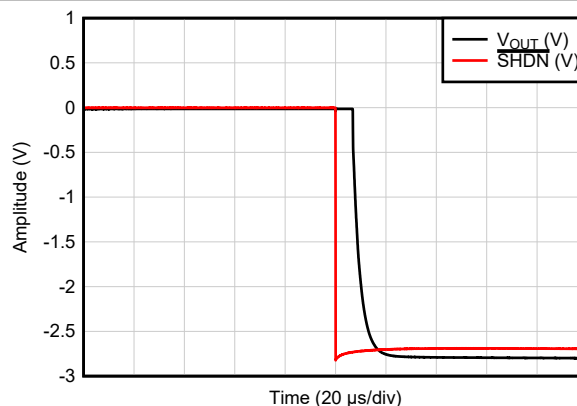
图 6-44. 放大器禁用响应
