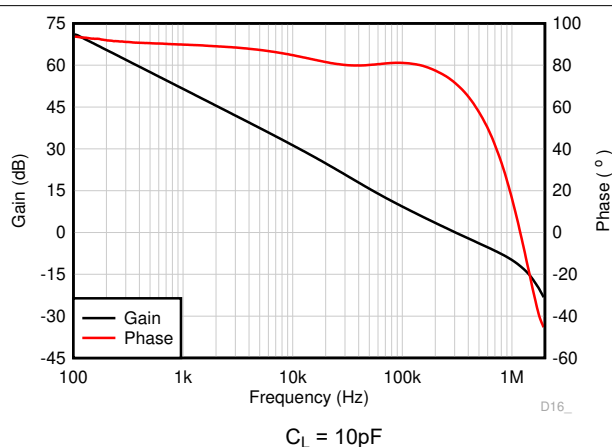
图 6-11. 开环增益和相位与频率间的关系
