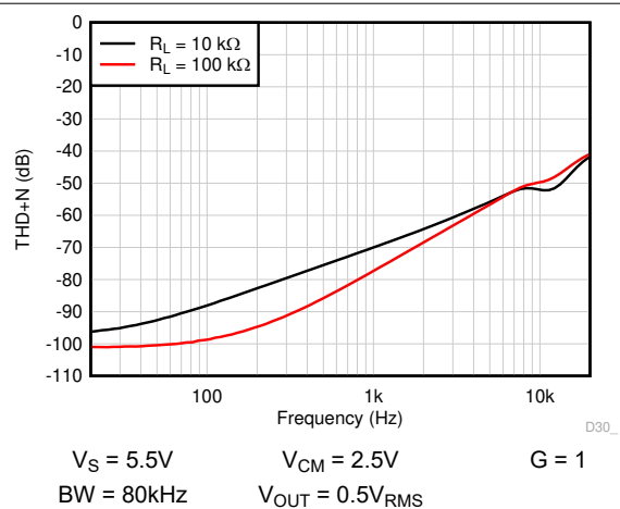
图 6-23. THD+N 与频率间的关系
