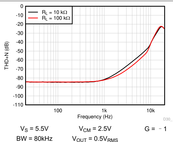
图 6-24. THD+N 与频率间的关系
