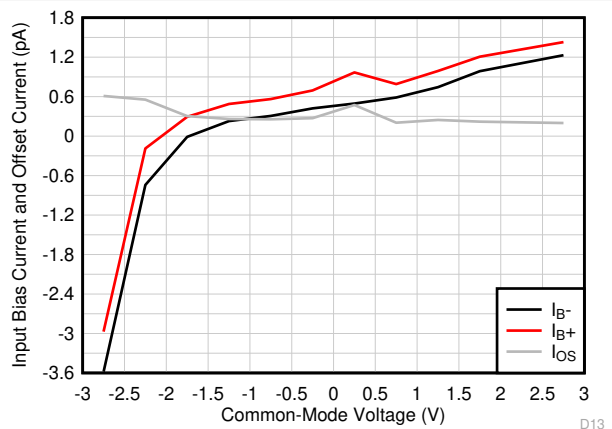
图 6-9. I_B 和 I_{OS} 与共模电压间的关系
