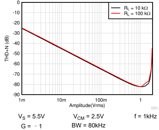
图 6-26. THD + N 与幅度间的关系
