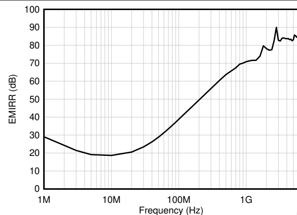
图 6-45. 以同相输入为基准的电磁干扰抑制比 (EMIRR+) 与频率间的关系
