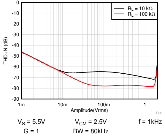
图 6-25. THD + N 与幅度间的关系
