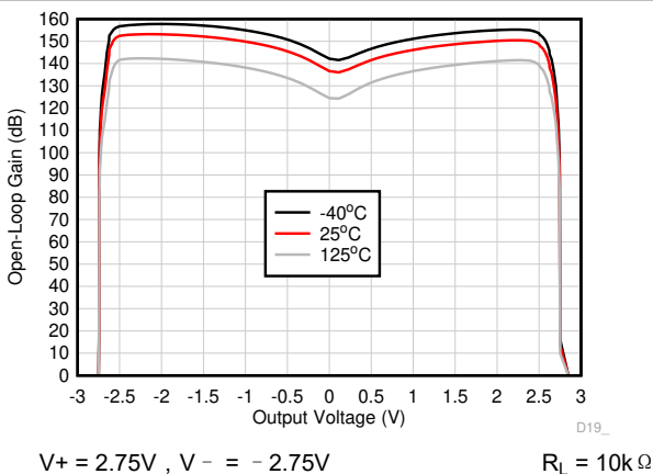
图 6-13. 开环增益与输出电压间的关系
