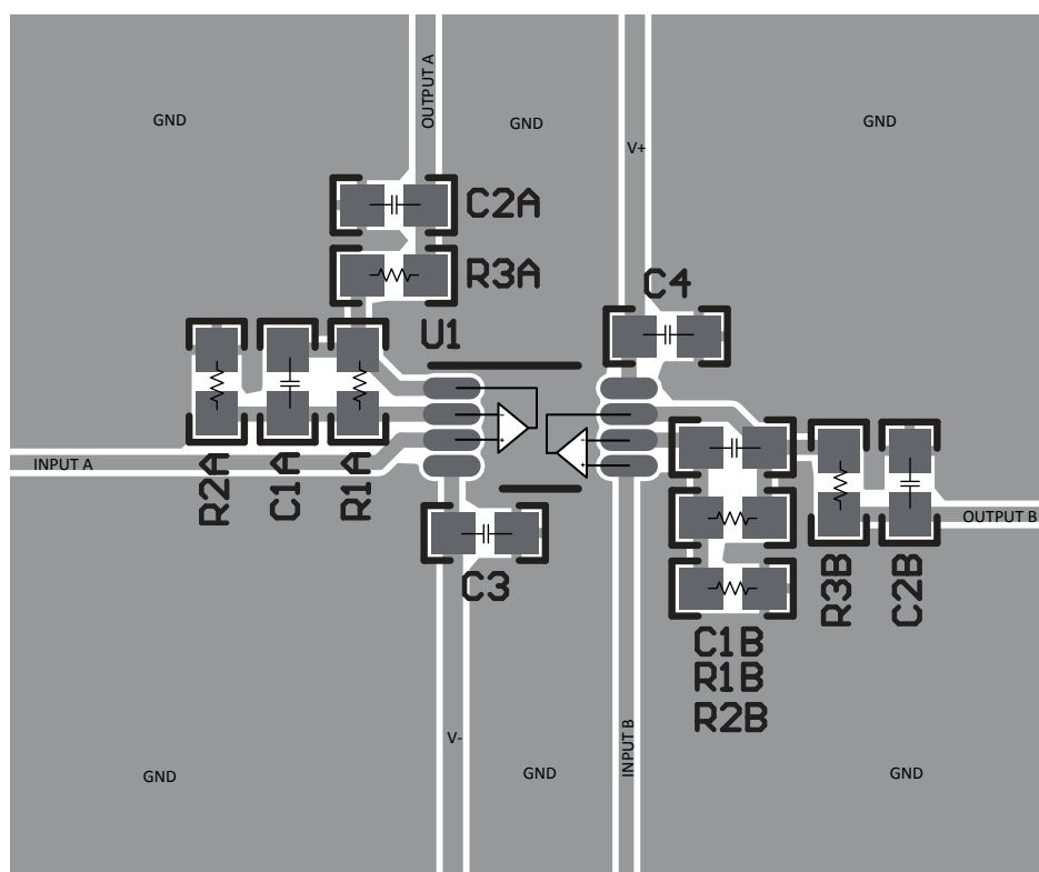
图 8-5. VSSOP-8 (DGK) 封装的布局示例
