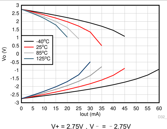
图 6-15. 输出电压与输出电流间的关系 ( 爪形 )
