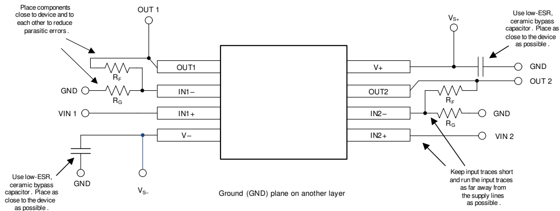
图 8-4. 布局示例
