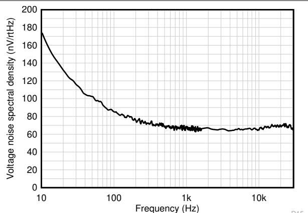
图 6-22. 输入电压噪声频谱密度
