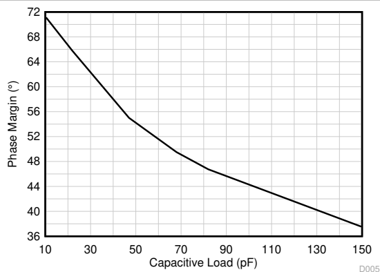
图 6-31. 相位裕度与容性负载间的关系
