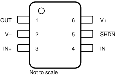
图 5-5. TLV9041S DBV 封装 6 引脚 SOT-23 顶视图
