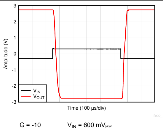
图 6-33. 过载恢复
