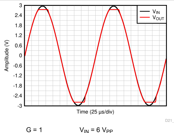
图 6-32. 无相位反转
