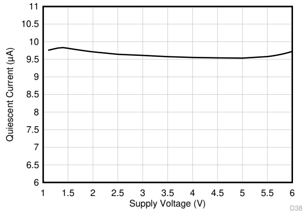
图 6-27. 静态电流与电源电压间的关系
