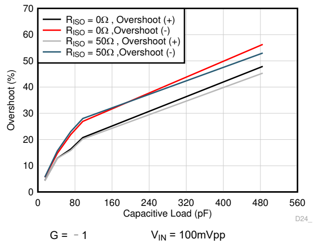
图 6-30. 小信号过冲与容性负载间的关系
