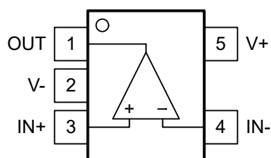
图 4-2. TLV9021、TLV9031 DCK 和 DBV 封装
