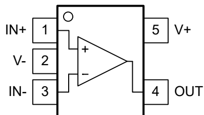
图 4-1. TLV9020、TLV9030 DCK 和 DBV 封装
