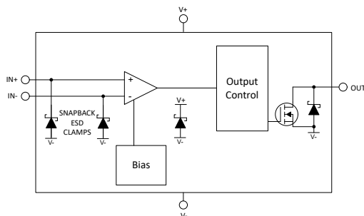
TLV902x 方框图
