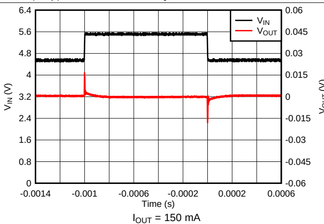
图 14. Line Transient
