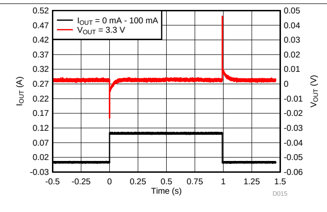
图 16. Load Transient
