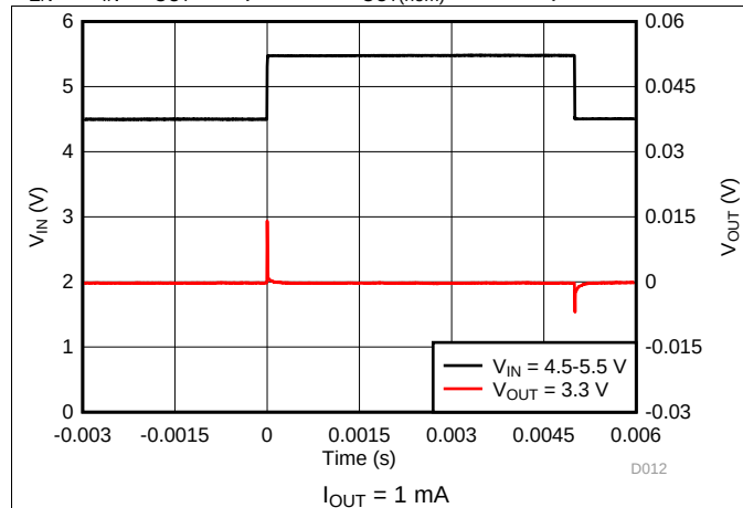
图 13. Line Transient
