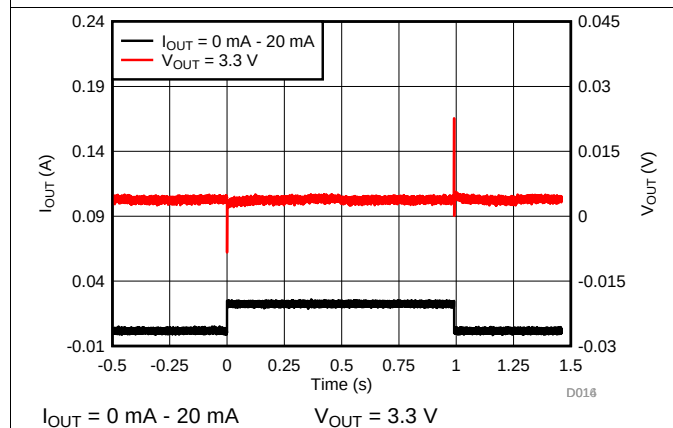
图 15. Load Transient
