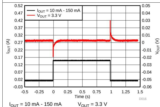
图 17. Load Transient
