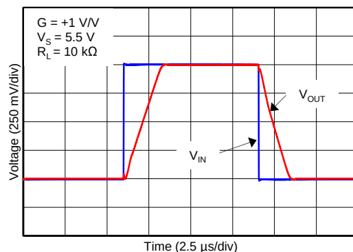
Figure 14. 小信号脉冲响应 (最大供电电压)
