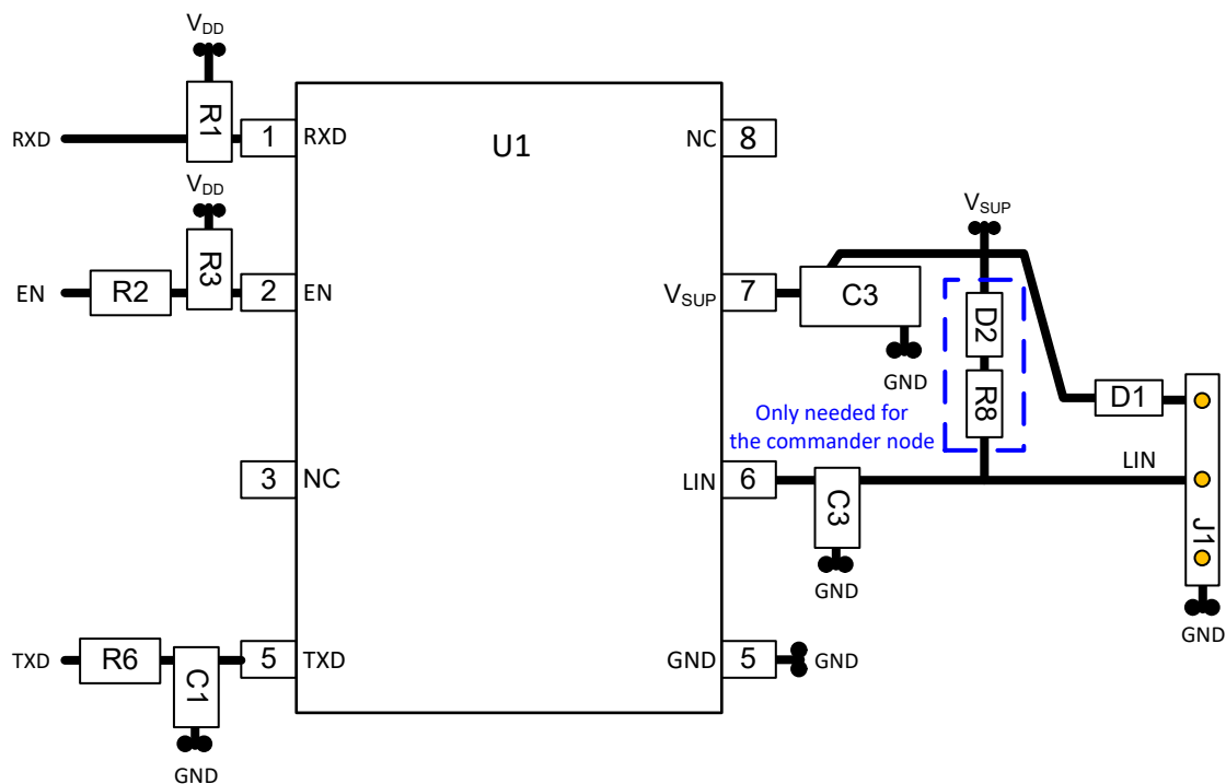
图 12-1. Layout Example
