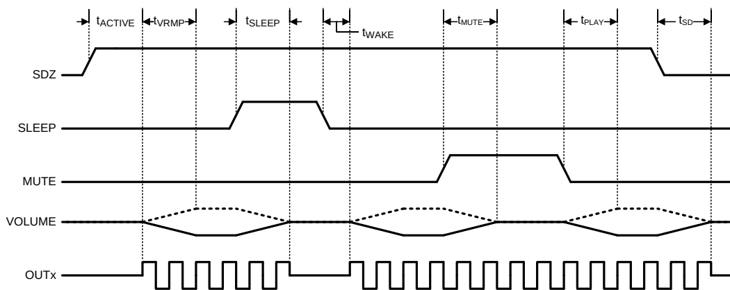
图 4. Mode Timing
