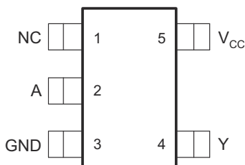
图 4-1. DBV 5 引脚 SOT-23 顶视图
