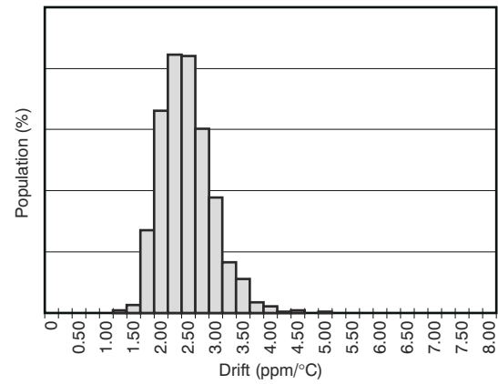
图 6-2. 温漂
