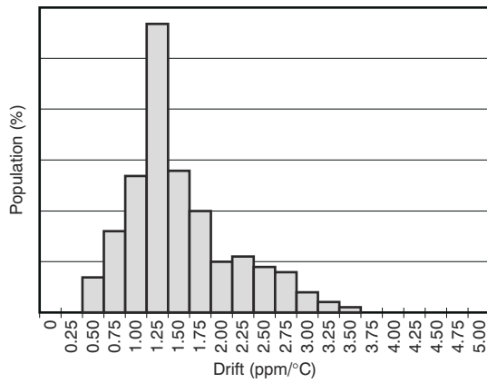
图 6-1. 温漂
