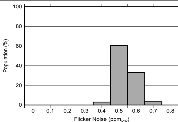
图 6-45. 0.1Hz 至 10Hz 电压噪声分布 ( C_{NR} = \text{开路} )
