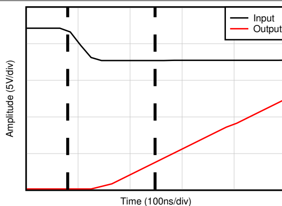
图 5-36. 负过载恢复
