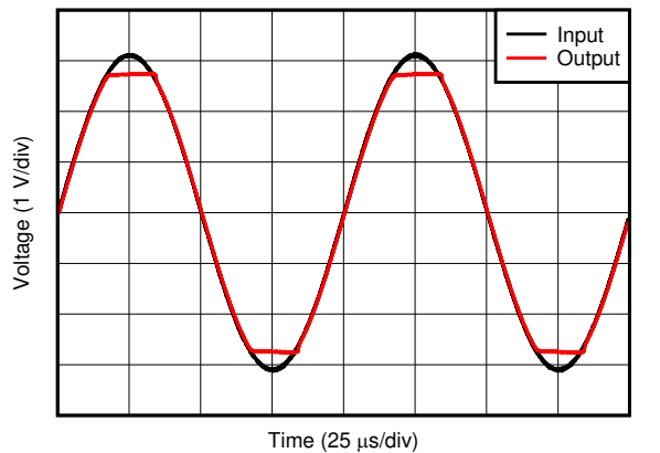
图 7-29. No Phase Reversal
