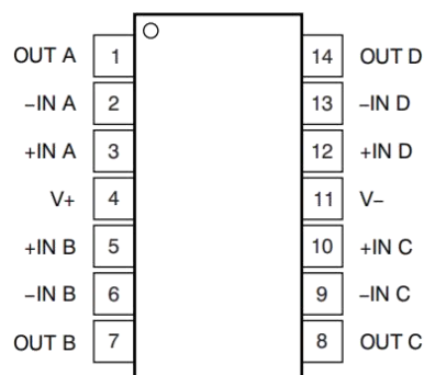
封装：OPA4333 14 引脚 TSSOP 俯视图
