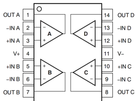
封装：OPA4333 14 引脚 SOP 俯视图
