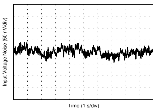
OPAx210 0.1\text{Hz} 至 10\text{Hz} 噪声
