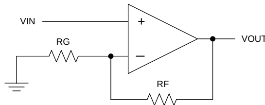
图 70. 原理图表示
