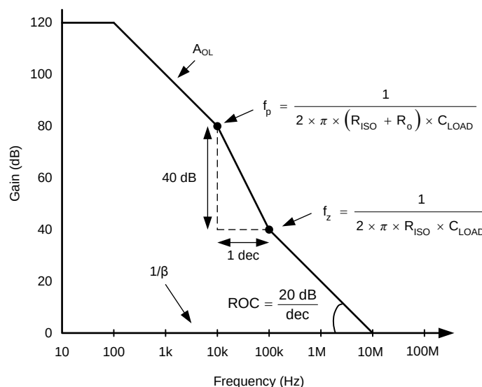
图 42. 具有 R_{ISO} 补偿的单位增益放大器
