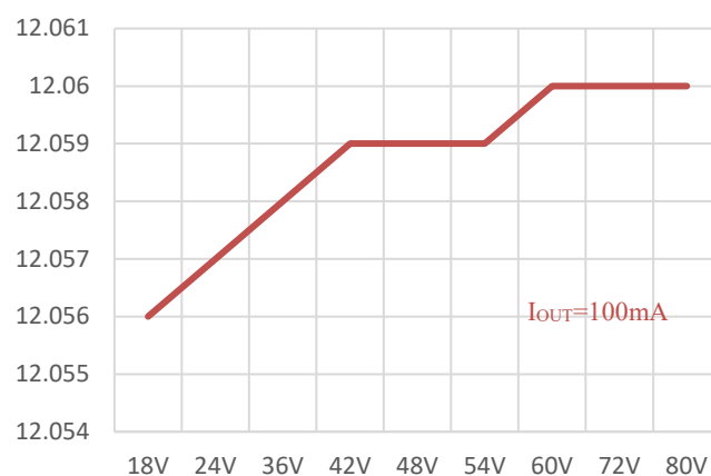
图2 线性调整
