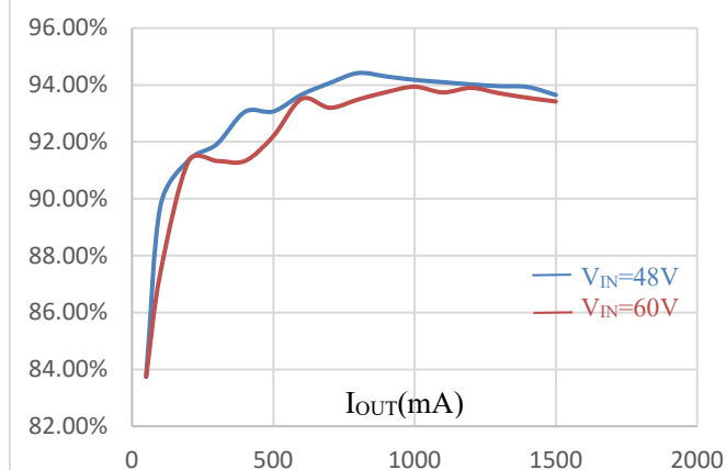
图1 效率曲线
