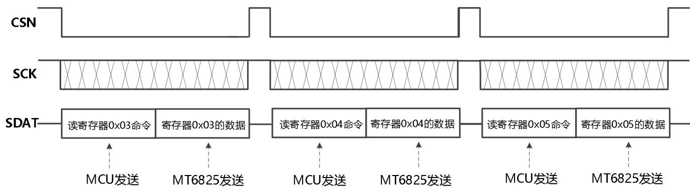
图-21：3线SPI单字节读角度模式
