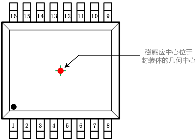
图-1: MT6825 TSSOP-16封装外观图
