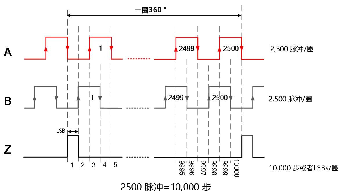
图-11: ABZ输出分辨率=2500 脉冲/圈
