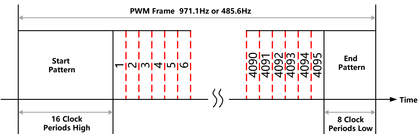
图-13: PWM输出
