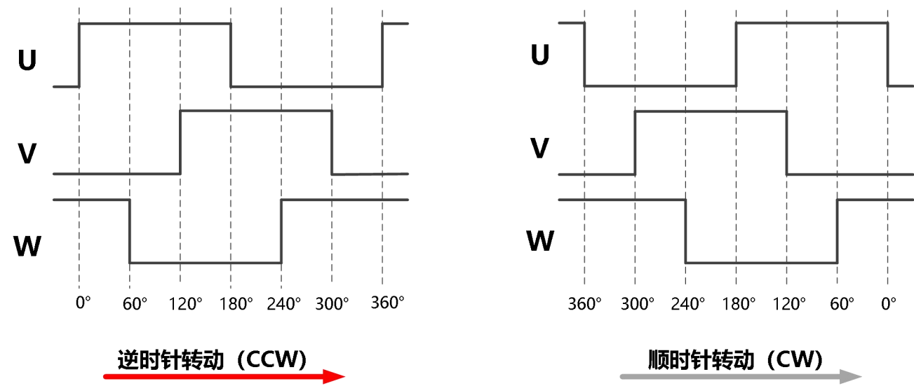
图-12: UVW输出波形
