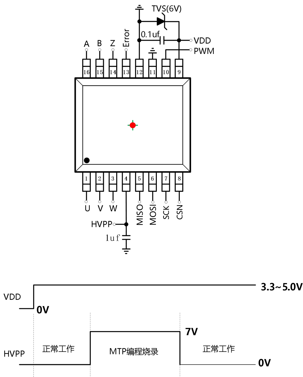
图-23: MTP编程
