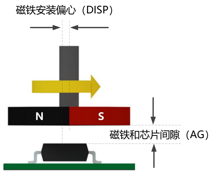
图-24: 磁铁安装
