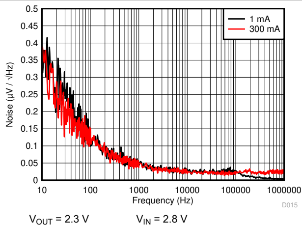
图 6-15. Noise Density
