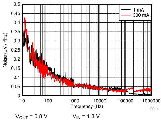
图 6-14. Noise Density
