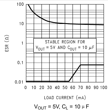
图 7-4. 5V, 10 \mu F ESR Curves (Legacy Chip)
