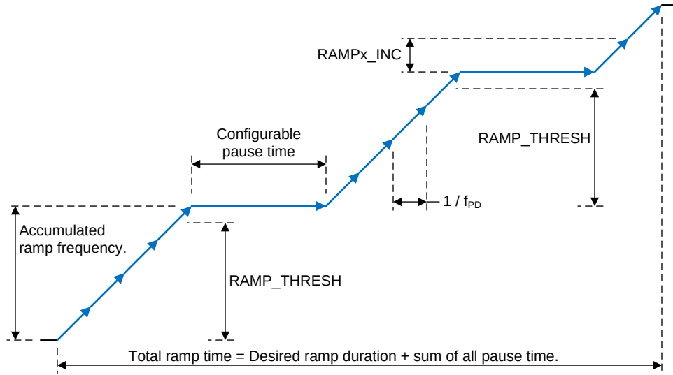
图 162. Auto Ramp Waveform
