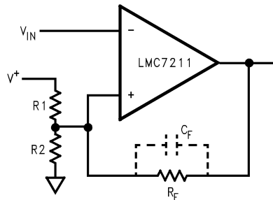
图 5-2. 磁滞正反馈
