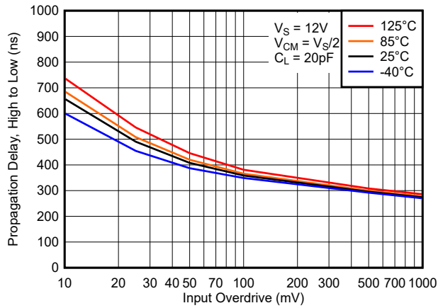
图 4-9. 传播延迟, 从高电平到低电平, 12V
