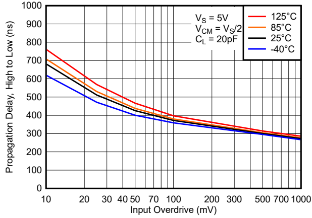
图 4-7. 传播延迟, 从高电平到低电平, 5V
