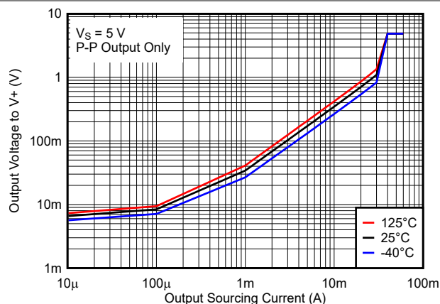
图 4-4. 输出电压与输出拉电流间的关系，5V
