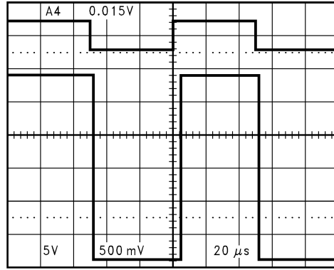
图 5-1. 即使在 2.7V 的低电源电压下，超过电源电压的输入信号也不会在输出端产生相位反转
