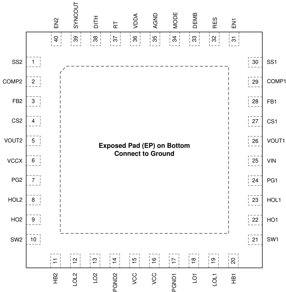
图 7-1. 封装 ( 顶视图 )
