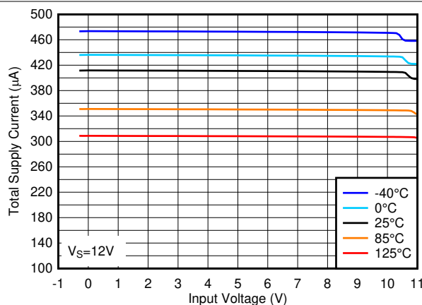
图 5-5. 12V 下总电源电流与输入电压之间的关系
