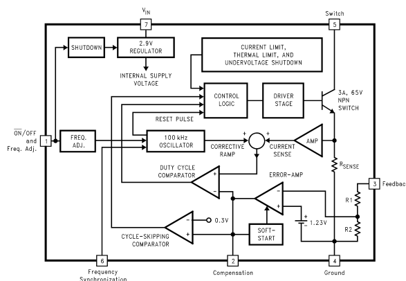
方框图
