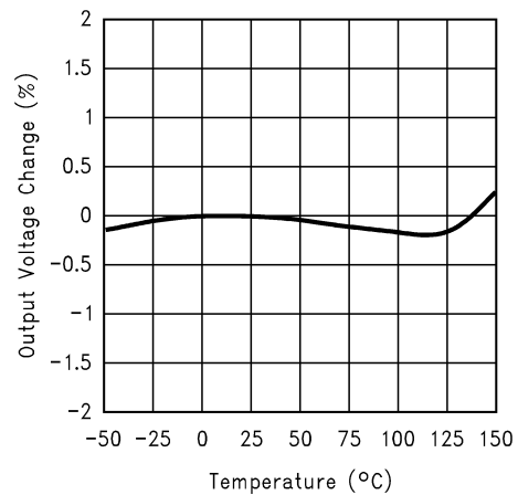
图 7-6. 温度稳定性
