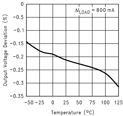
图 7-3. 负载调整率
