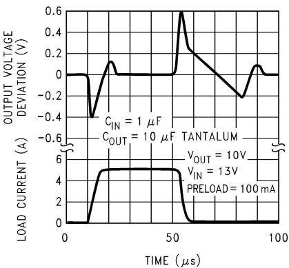
图 5-8. LM1084-ADJ Load Transient Response
