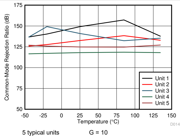
图 7-15. CMRR vs Temperature
