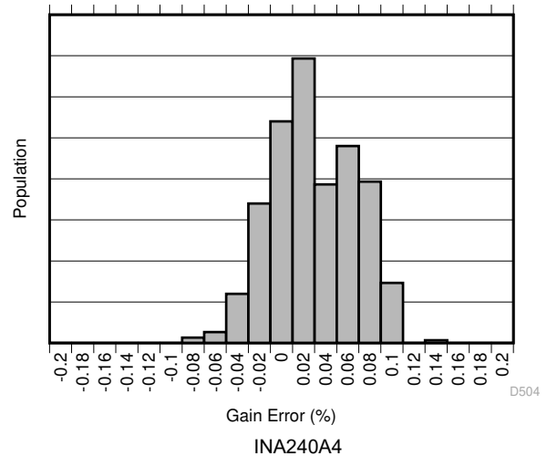
图 7-8. 增益误差产生分布图
