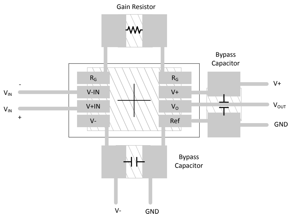
图 7-9. INA126 布局示例
