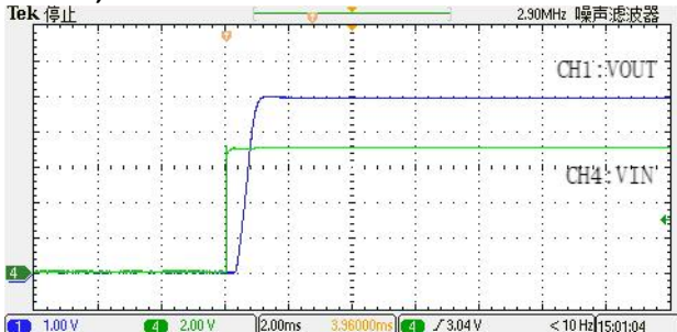
VIN=7V, VOUT=5V
